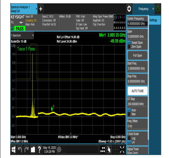
NTNV_N77-3450-3550_PC2_30_50_L_TID4_N/A _3000_6000_#1
