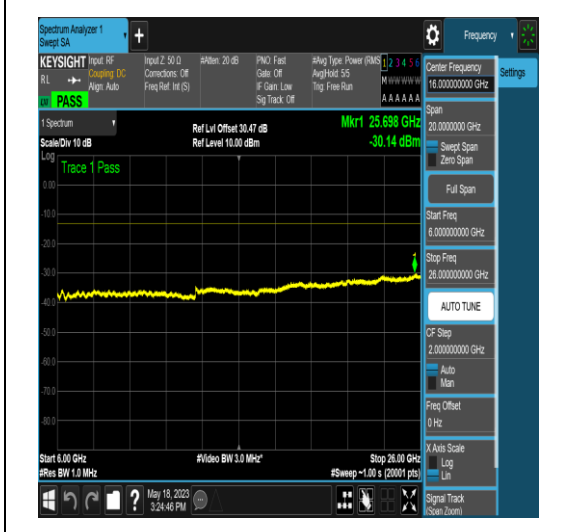
NTNV_N77-3450-3550_PC2_30_50_L_TID4_N/A _1000_3000_#1
