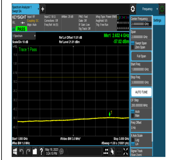
NTNV_N77-3450-3550_PC2_30_50_L_TID4_N/A _1000_3000_#1
