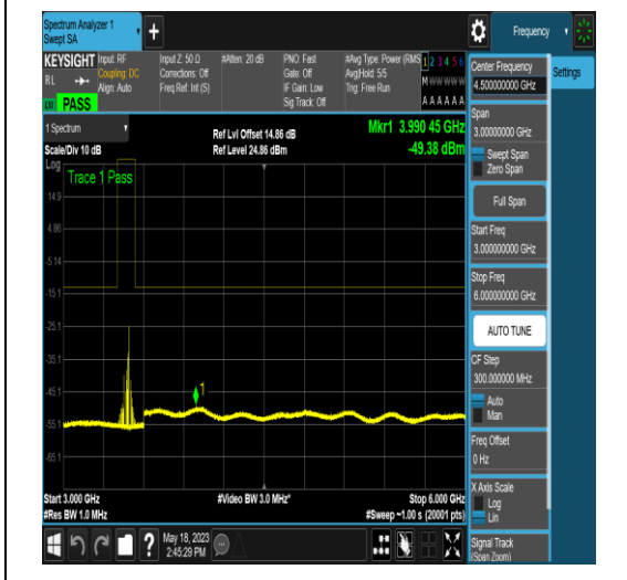
NTNV_N77-3450-3550_PC2_30_40_L_TID5_N/A _30_1000_#1
