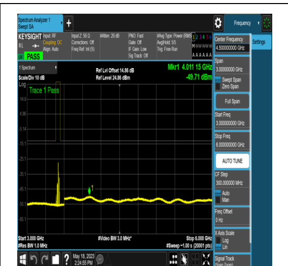
NTNV_N77-3450-3550_PC2_30_20_M_TID17_NV/ A_3000_6000_#1
