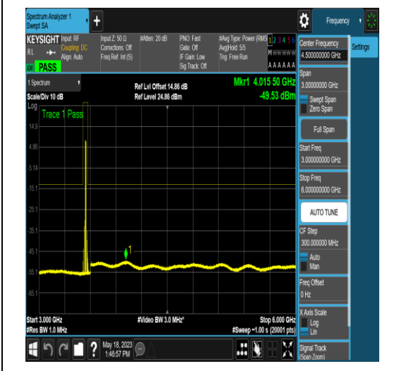
NTNV_N77-3450-3550_PC2_30_15_H_TID6_N/A _3000_6000_#1
