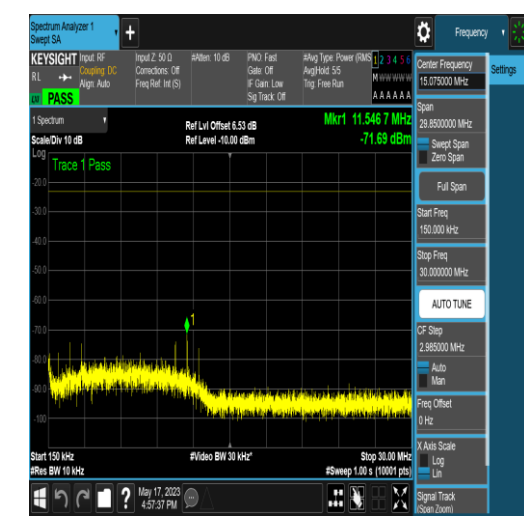
NTNV_N71_PC3_15_15_L_TID6_N/A_0.15_30_# 1
