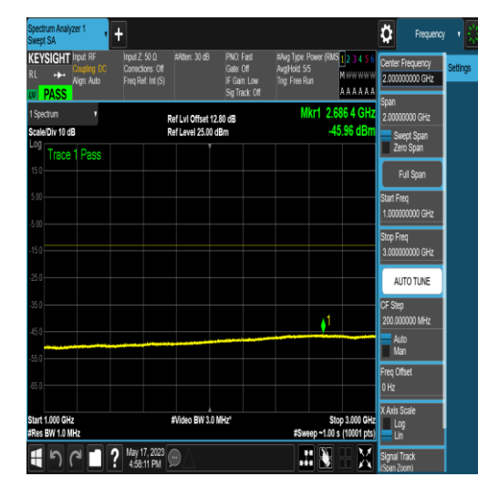
NTNV_N71_PC3_15_15_L_TID6_N/A_0.15_30_# 1
