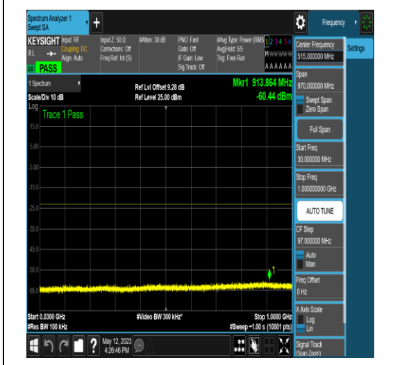
NTNV_N66_PC3_15_15_L_TID16_N/A_30_1000 _#1
