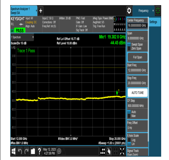
NTNV_N66_PC3_15_15_L_TID16_N/A_1000_30 00_#1
