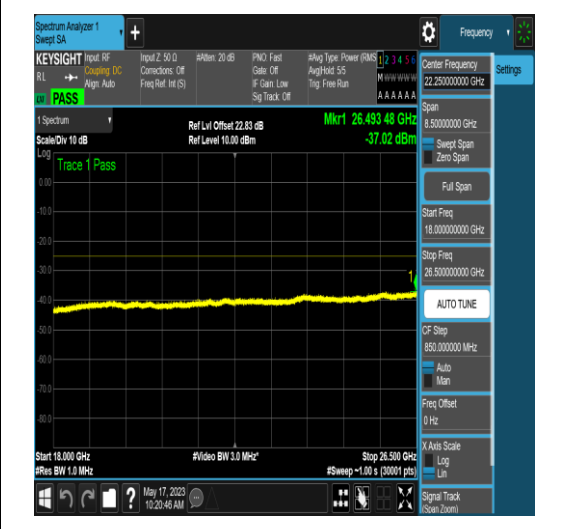
NTNV_N41_PC2_30_90_H_TID18_N/A_18000_2 6500_#1
