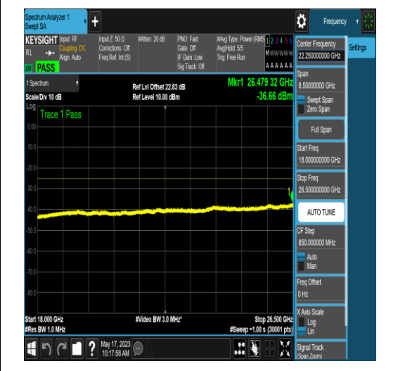
NTNV_N41_PC2_30_90_H_TID4_N/A_1000_300 0_#1
