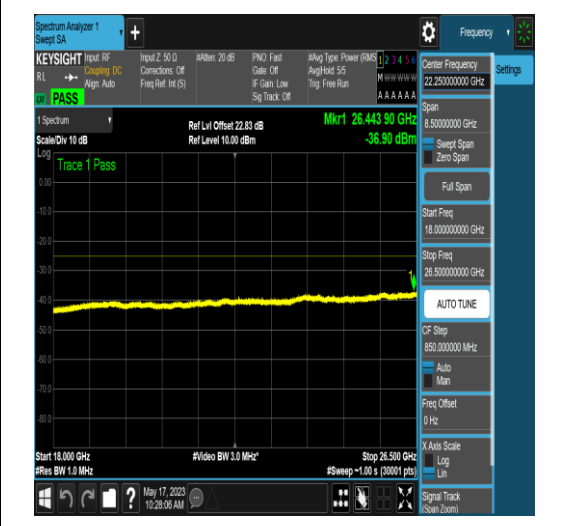
NTNV_N41_PC2_30_100_L_TID5_N/A_18000_26500_#1
