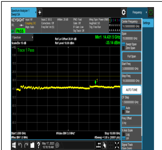
NTNV_N41_PC2_30_90_H_TID6_N/A_3000_180 00_#1
