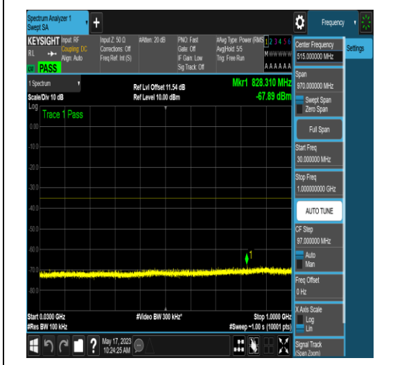
NTNV_N41_PC2_30_100_L_TID6_N/A_30_1000_#1
