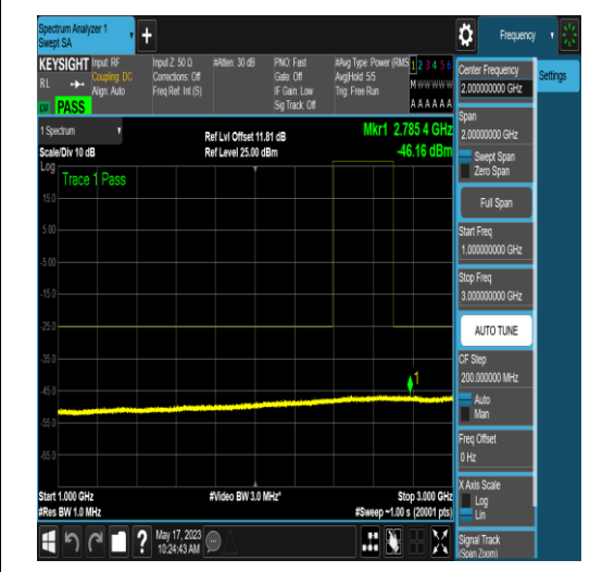
NTNV_N41_PC2_30_100_L_TID6_N/A_1000_3000_#1
