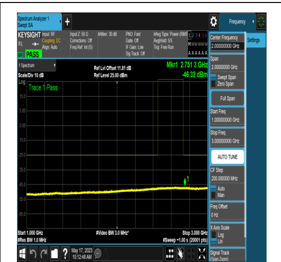
NTNV_N41_PC2_30_90_M_TID16_N/A_1000_30 00_#1
