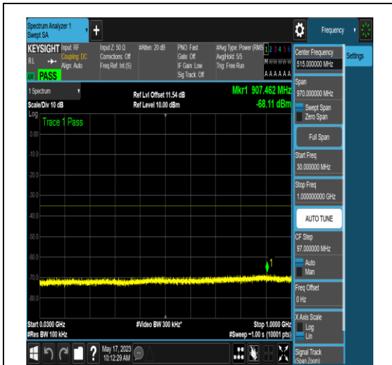
NTNV_N41_PC2_30_90_M_TID16_N/A_30_1000 _#1
