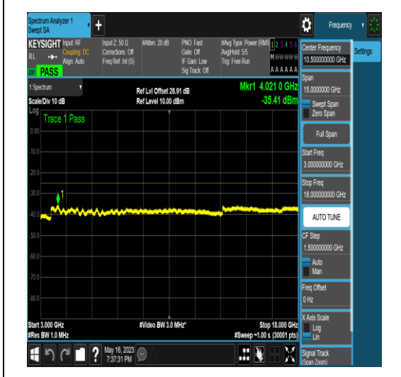
NTNV_N41_PC2_30_60_L_TID16_N/A_30_1000_#1
