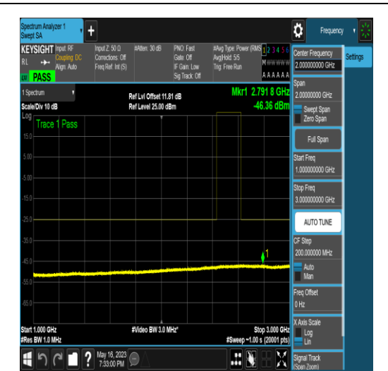
NTNV_N41_PC2_30_60_L_TID4_N/A_1000_300
