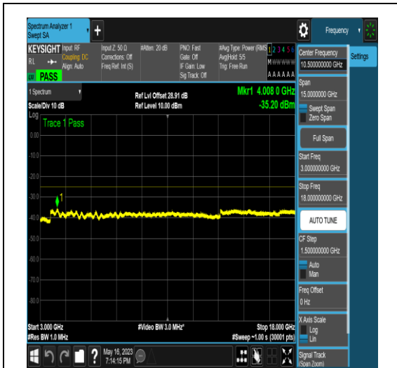
NTNV_N41_PC2_30_50_M_TID6_N/A_3000_180 00_#1
