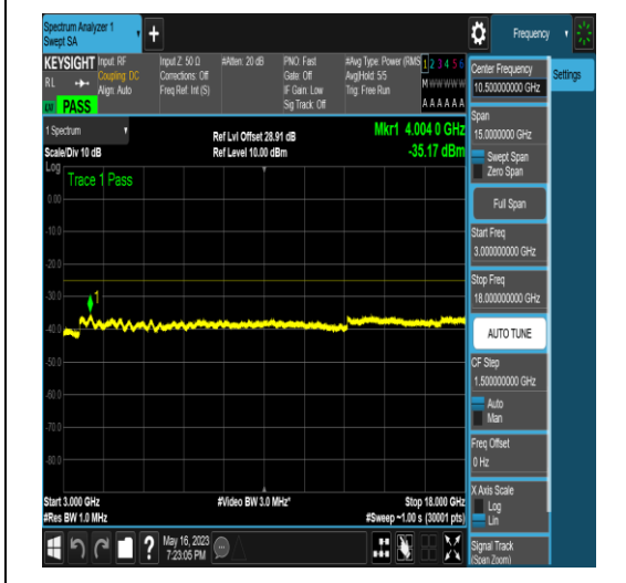
NTNV_N41_PC2_30_50_H_TID6_N/A_30_1000_#1
