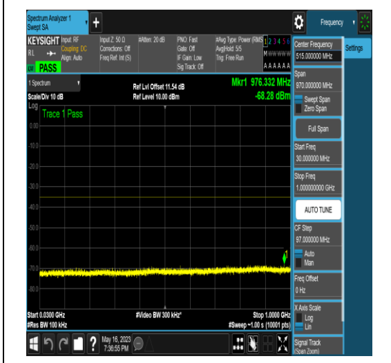
NTNV_N41_PC2_30_60_L_TID16_N/A_30_1000_#1
