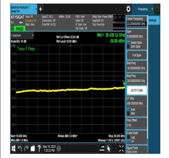
NTNV_N41_PC2_30_50_H_TID6_N/A_1000_300_0_#1
