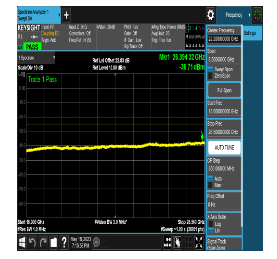
NTNV_N41_PC2_30_50_M_TID4_N/A_1000_300 0_#1
