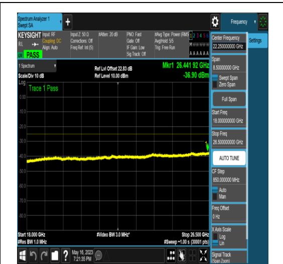
NTNV_N41_PC2_30_50_M_TID17_N/A_18000_2 6500_#1
