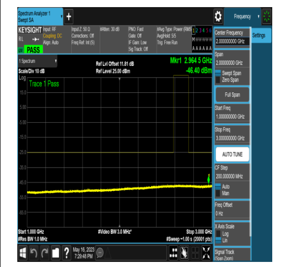
NTNV_N41_PC2_30_50_H_TID17_N/A_1000_3000_#1
