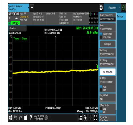
NTNV_N41_PC2_30_50_H_TID5_N/A_18000_26_500_#1
