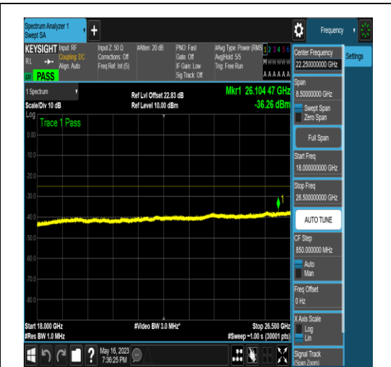
NTNV_N41_PC2_30_60_L_TID18_N/A_18000_2_6500_#1
