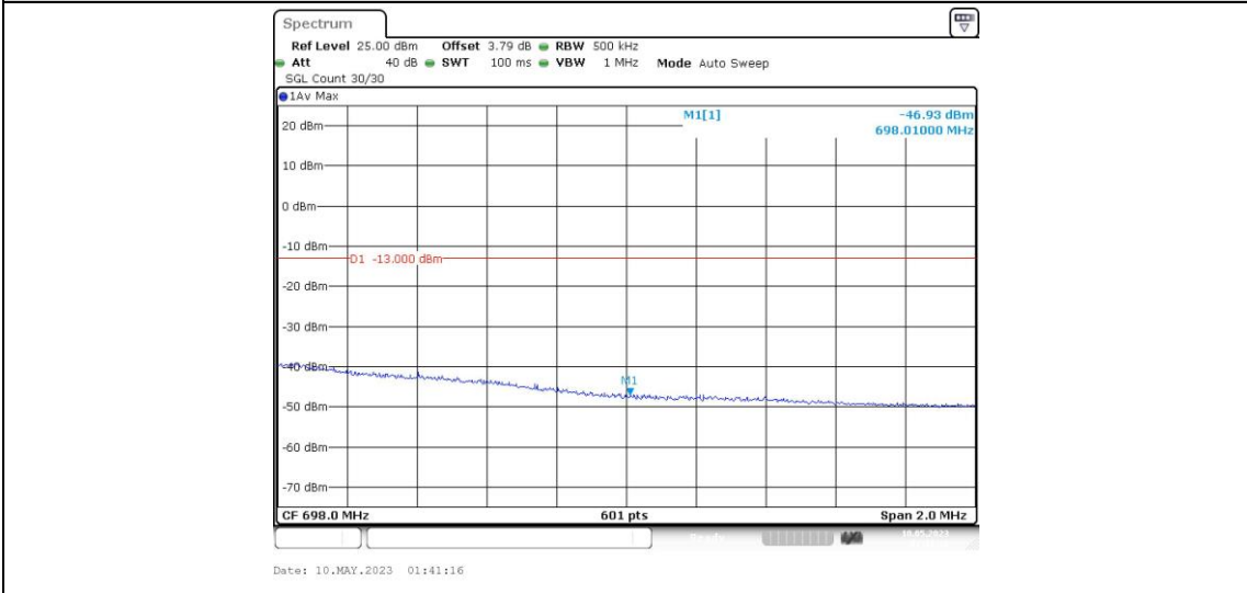
Band71-20MHz-16QAM-133372-1RB#99
