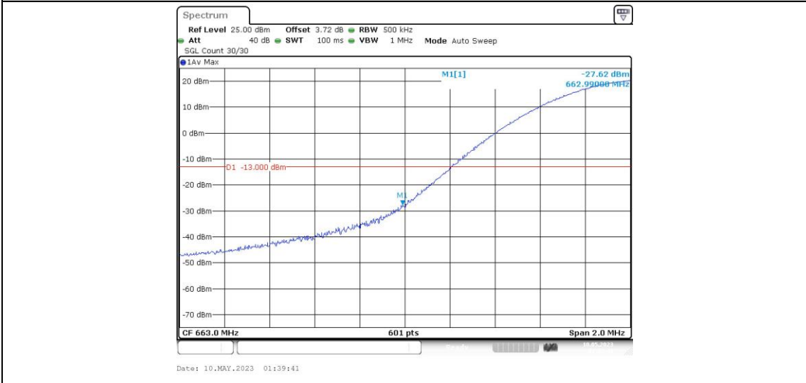
Band71-20MHz-QPSK-133222-1RB#99
