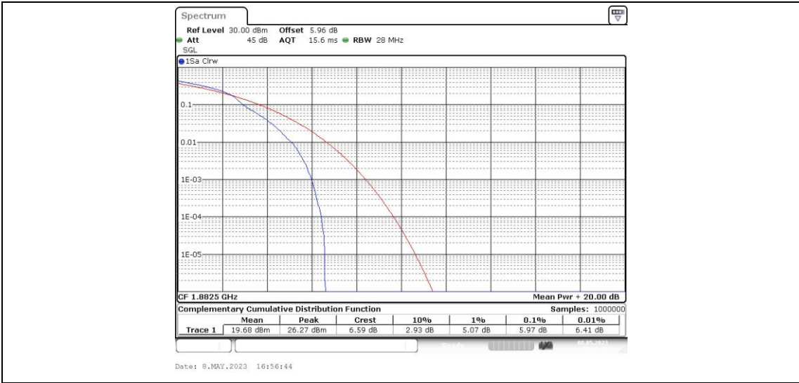
Band25-10MHz-16QAM-26365-50RB#0
