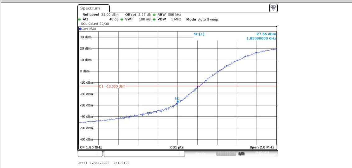
Band2-20MHz-16QAM-18700-1RB#99
