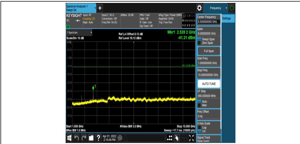
Band26-3MHz-QPSK-27025-1RB#0-Range4:1000~10000MHz
