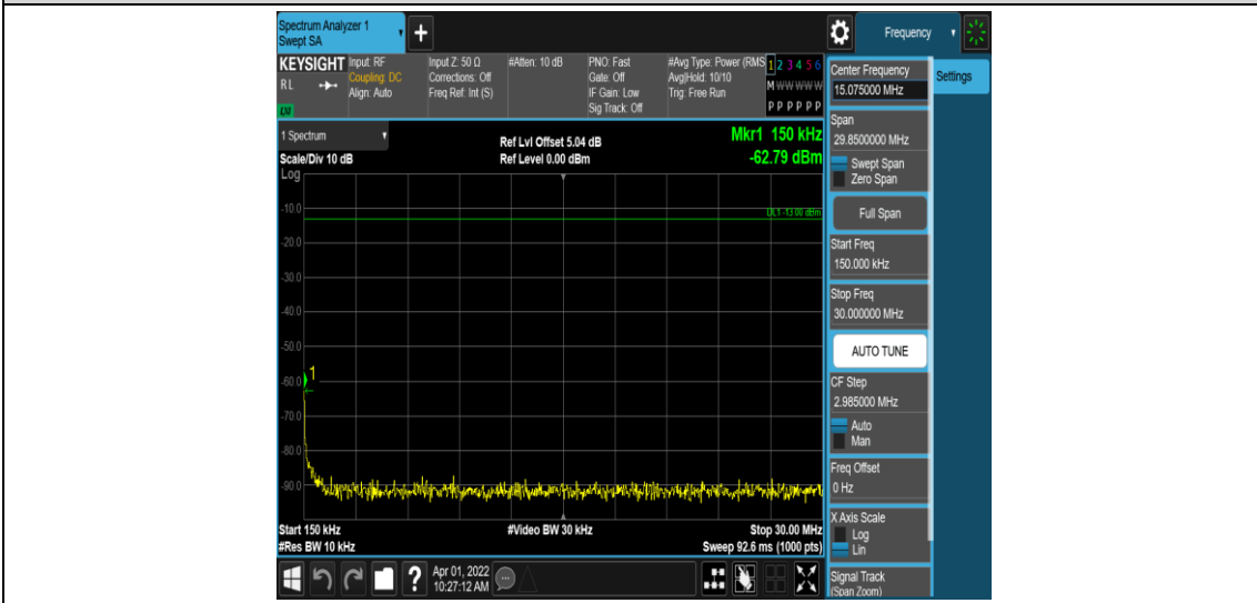
Band71-10MHz-QPSK-133422-1RB#0-Range2:0.15~30MHz
