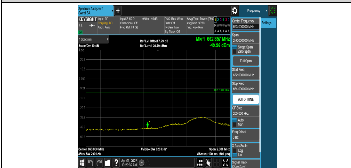
Band71-10MHz-QPSK-133172-1RB#49
