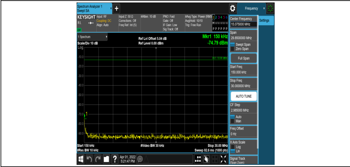
Band41-15MHz-QPSK-39725-1RB#0-Range2:0.15~30MHz
