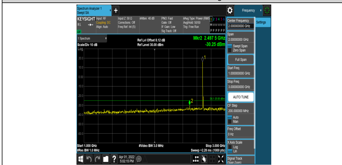
Band41-10MHz-QPSK-41540-1RB#0-Range4:1000~3000MHz
