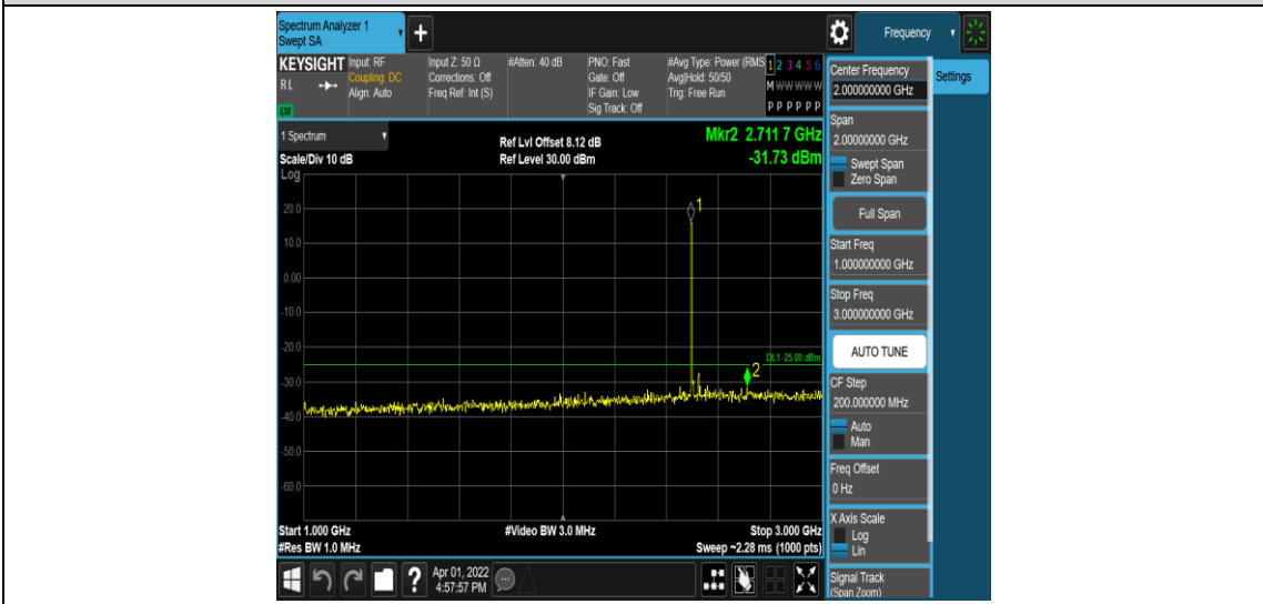
Band41-10MHz-QPSK-39700-1RB#0-Range4:1000~3000MHz
