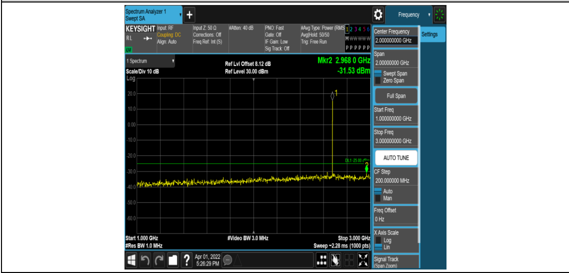
Band41-15MHz-QPSK-41515-1RB#0-Range4:1000~3000MHz
