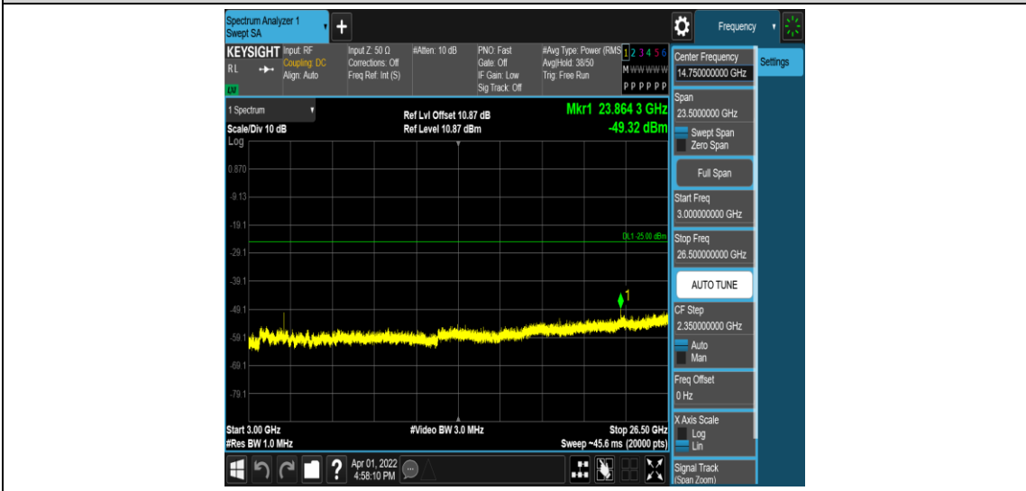
Band41-10MHz-QPSK-39700-1RB#0-Range5:3000~26500MHz
