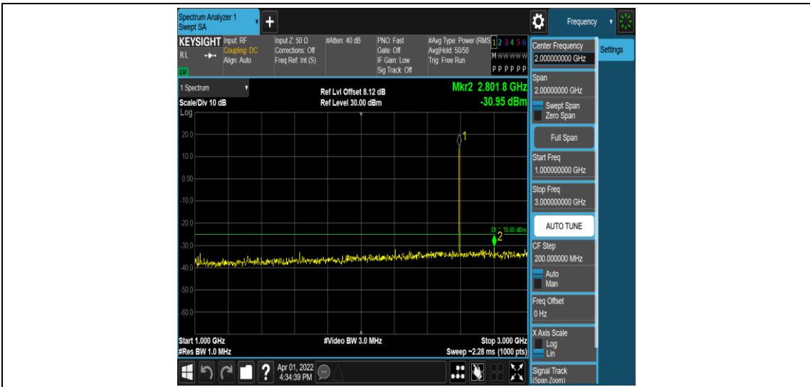
Band41-5MHz-QPSK-40620-1RB#0-Range4:1000~3000MHz
