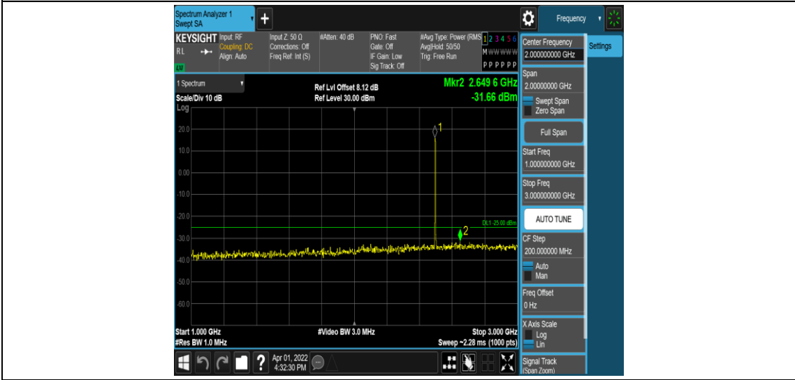
Band41-5MHz-QPSK-39675-1RB#0-Range4:1000~3000MHz
