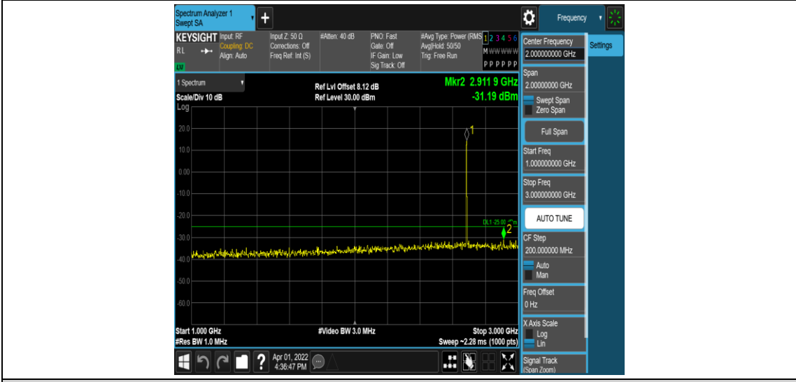
Band41-5MHz-QPSK-41565-1RB#0-Range4:1000~3000MHz
