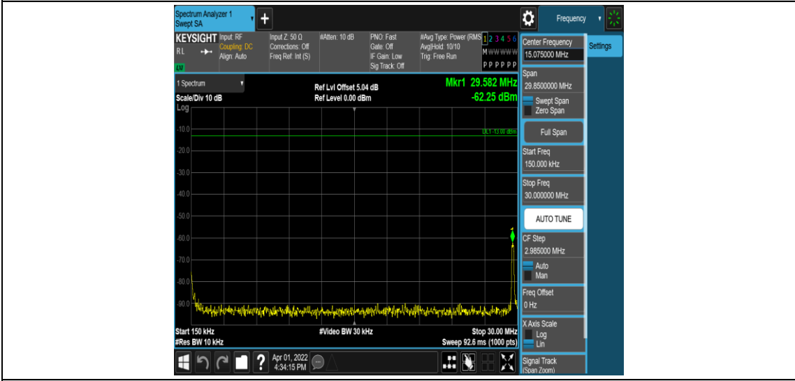
Band41-5MHz-QPSK-40620-1RB#0-Range2:0.15~30MHz
