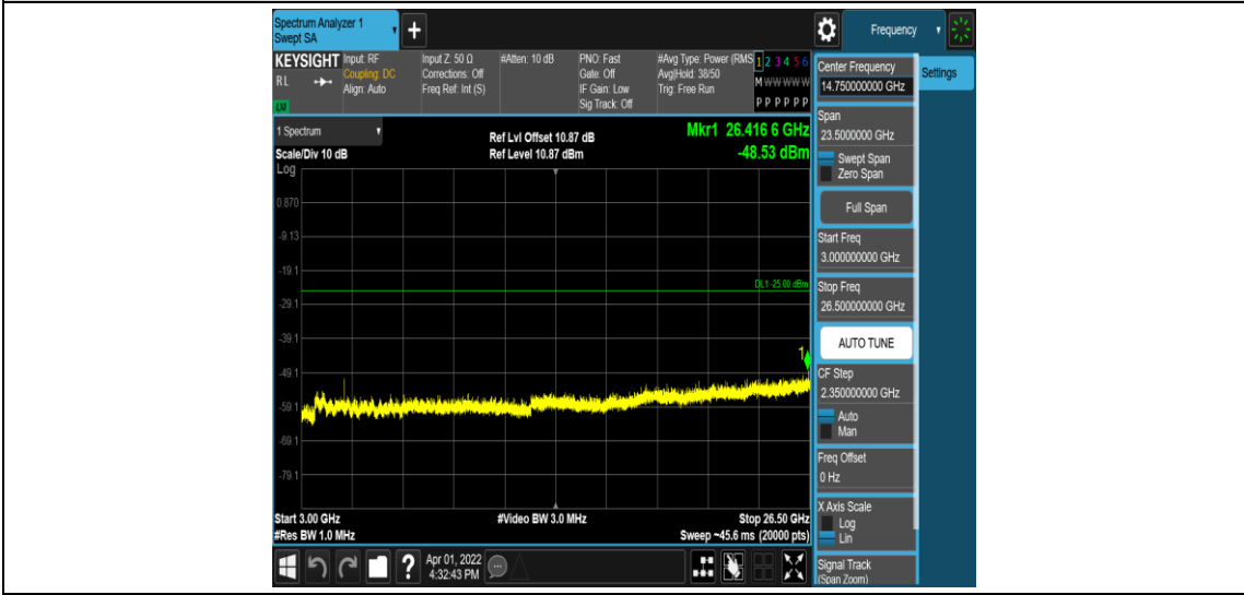
Band41-5MHz-QPSK-39675-1RB#0-Range5:3000~26500MHz
