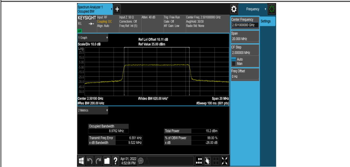
Band41-10MHz-QPSK-39700-50RB#0
