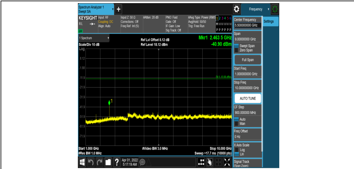
Band26-3MHz-QPSK-26775-1RB#0-Range4:1000~10000MHz
