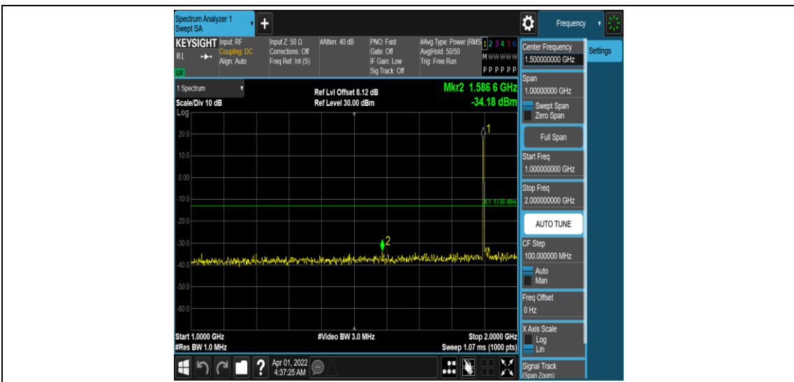
Band25-20MHz-QPSK-26590-1RB#0-Range4:1000~2000MHz
