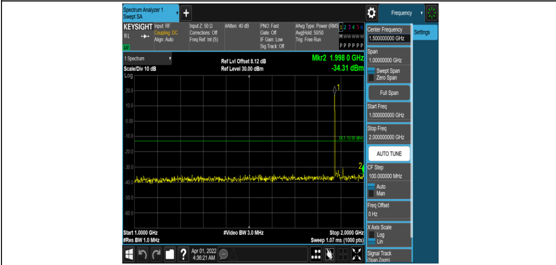
Band25-20MHz-16QAM-26365-1RB#0-Range4:1000~2000MHz
