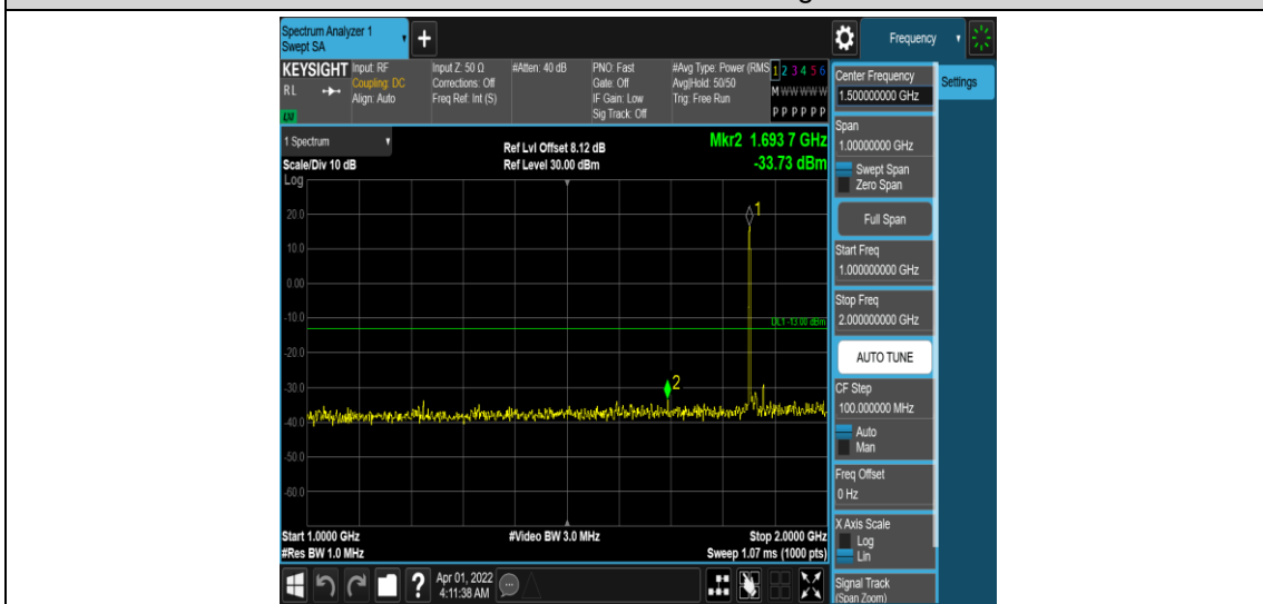
Band25-15MHz-QPSK-26115-1RB#0-Range4:1000~2000MHz
