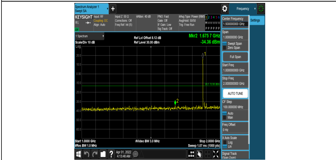
Band25-15MHz-QPSK-26365-1RB#0-Range4:1000~2000MHz
