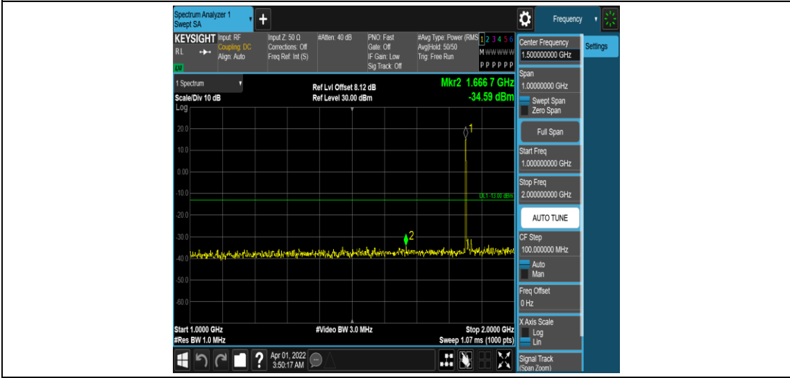
Band25-10MHz-QPSK-26090-1RB#0-Range4:1000~2000MHz
