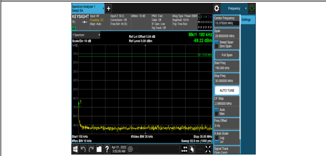
Band25-10MHz-QPSK-26365-1RB#0-Range2:0.15~30MHz
