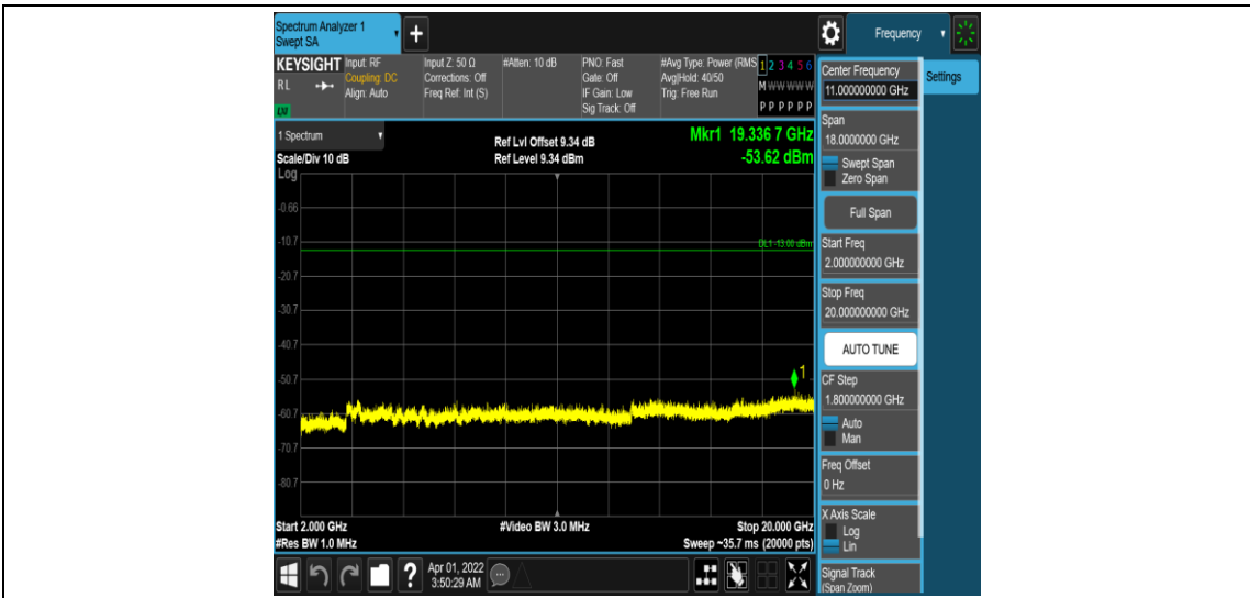
Band25-10MHz-QPSK-26090-1RB#0-Range5:2000~20000MHz
