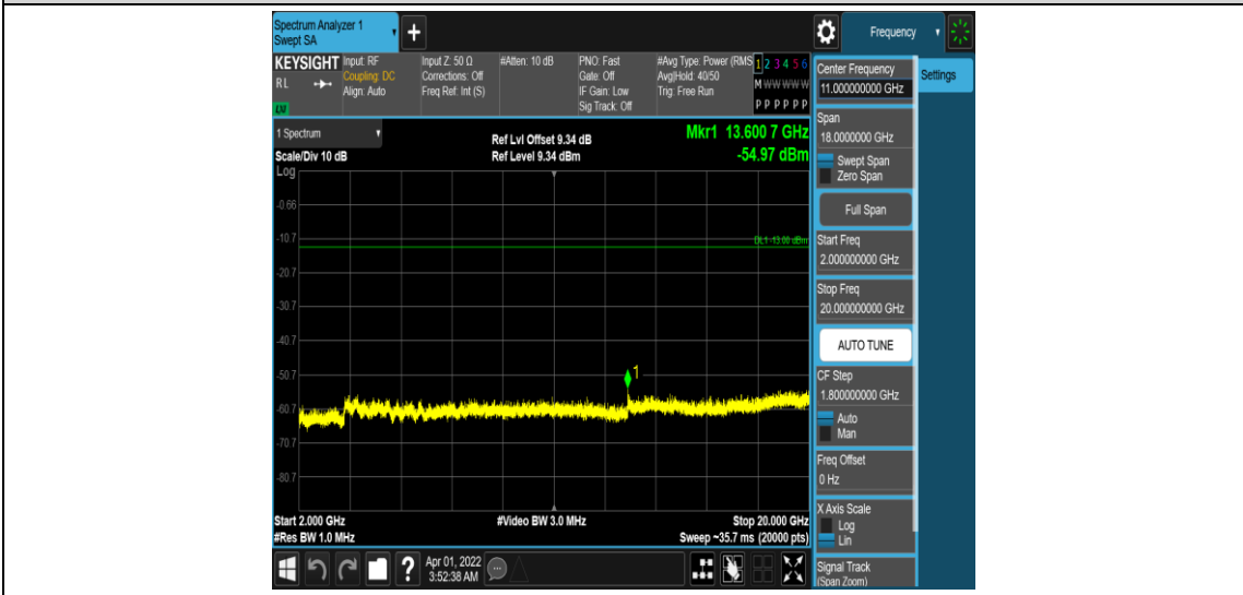
Band25-10MHz-QPSK-26365-1RB#0-Range5:2000~20000MHz
