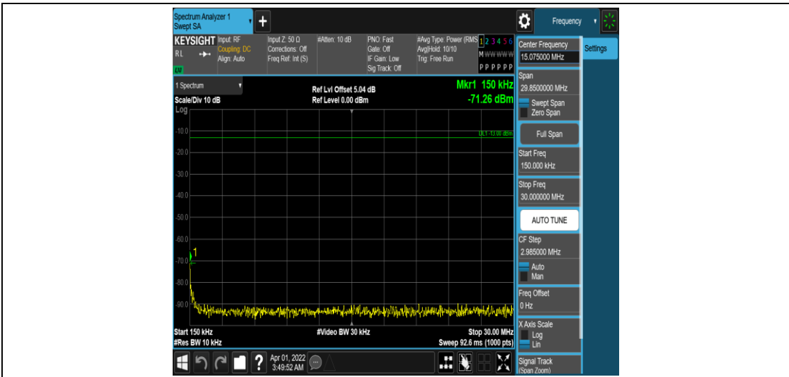
Band25-10MHz-QPSK-26090-1RB#0-Range2:0.15~30MHz
