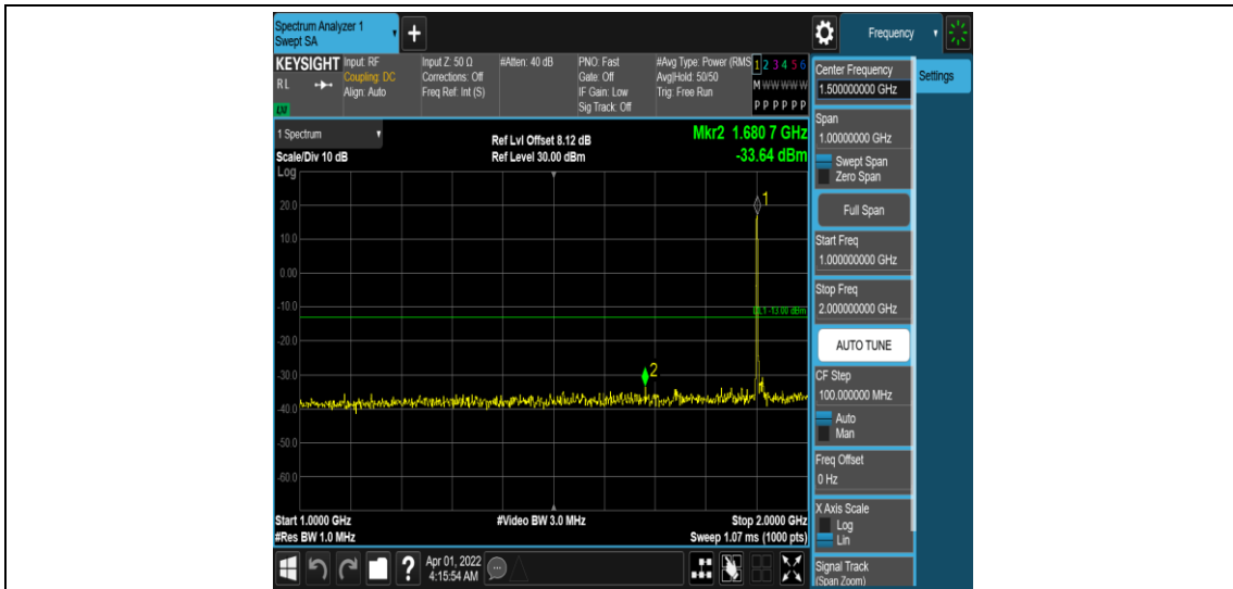
Band25-15MHz-QPSK-26615-1RB#0-Range4:1000~2000MHz
