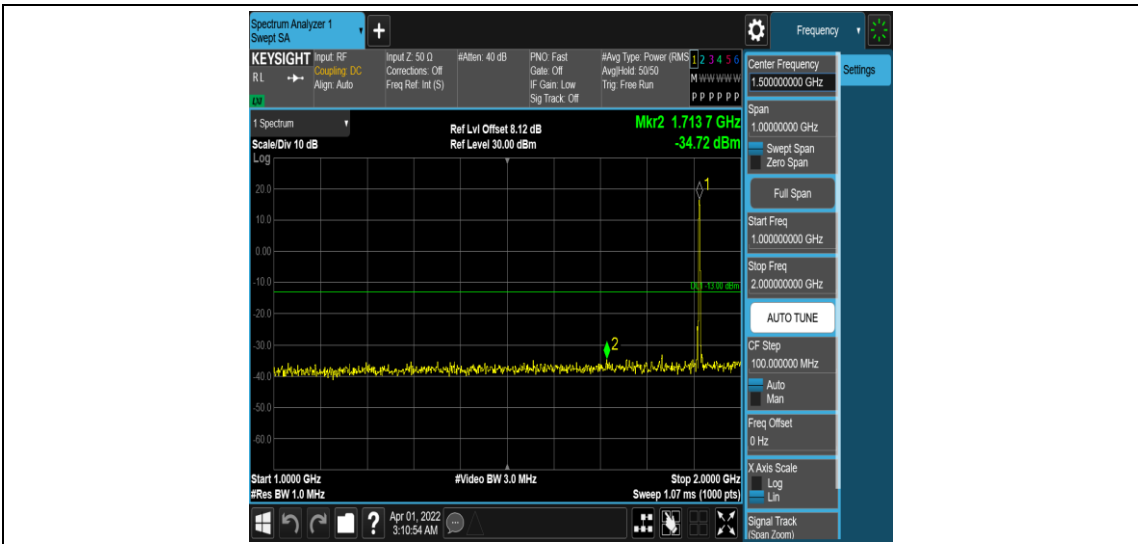
Band25-3MHz-QPSK-26675-1RB#0-Range4:1000~2000MHz
