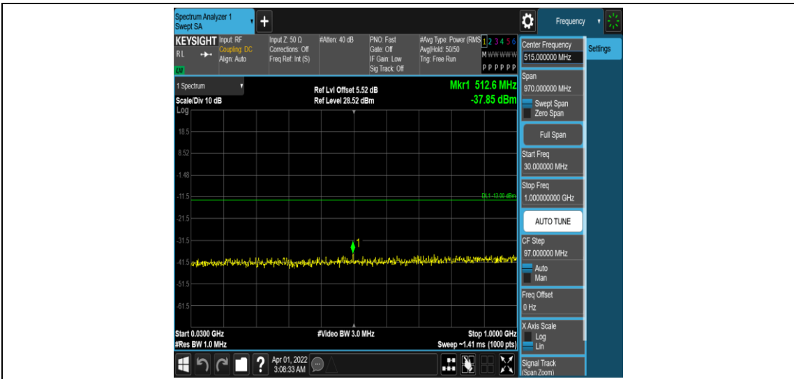
Band25-3MHz-QPSK-26365-1RB#0-Range3:30~1000MHz
