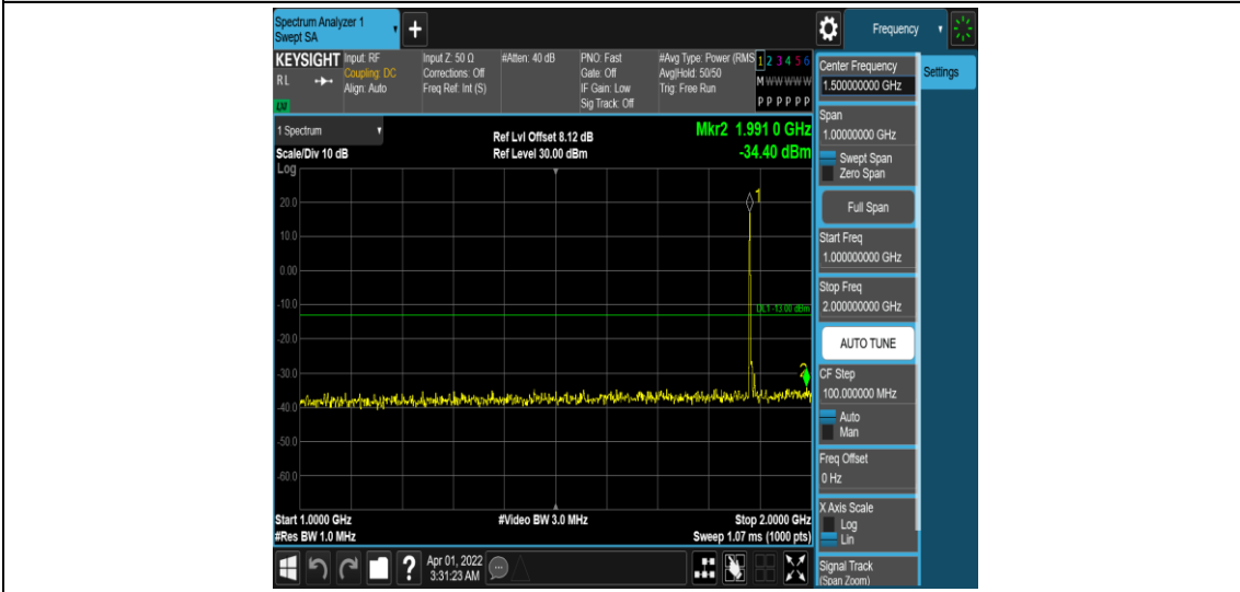
Band25-5MHz-QPSK-26365-1RB#0-Range4:1000~2000MHz
