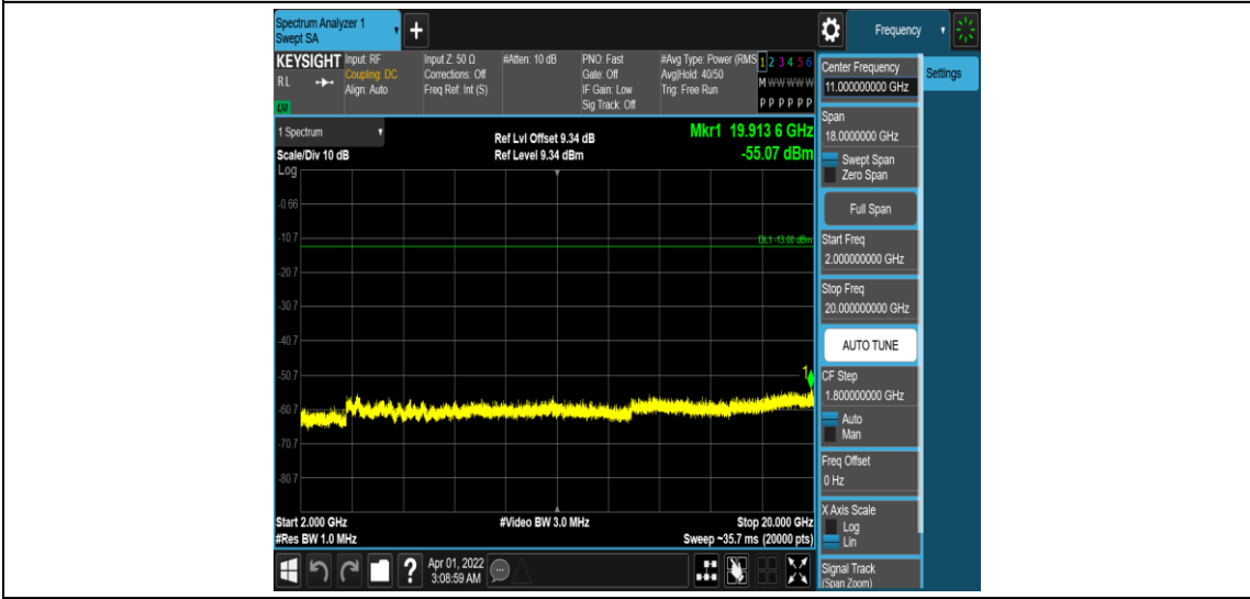
Band25-3MHz-QPSK-26365-1RB#0-Range5:2000~20000MHz
