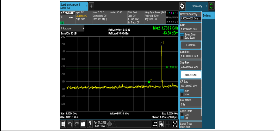
Band25-5MHz-QPSK-26065-1RB#0-Range4:1000~2000MHz
