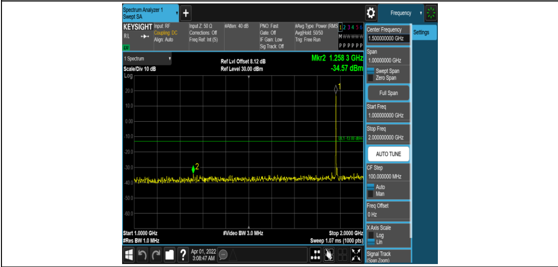
Band25-3MHz-QPSK-26365-1RB#0-Range4:1000~2000MHz
