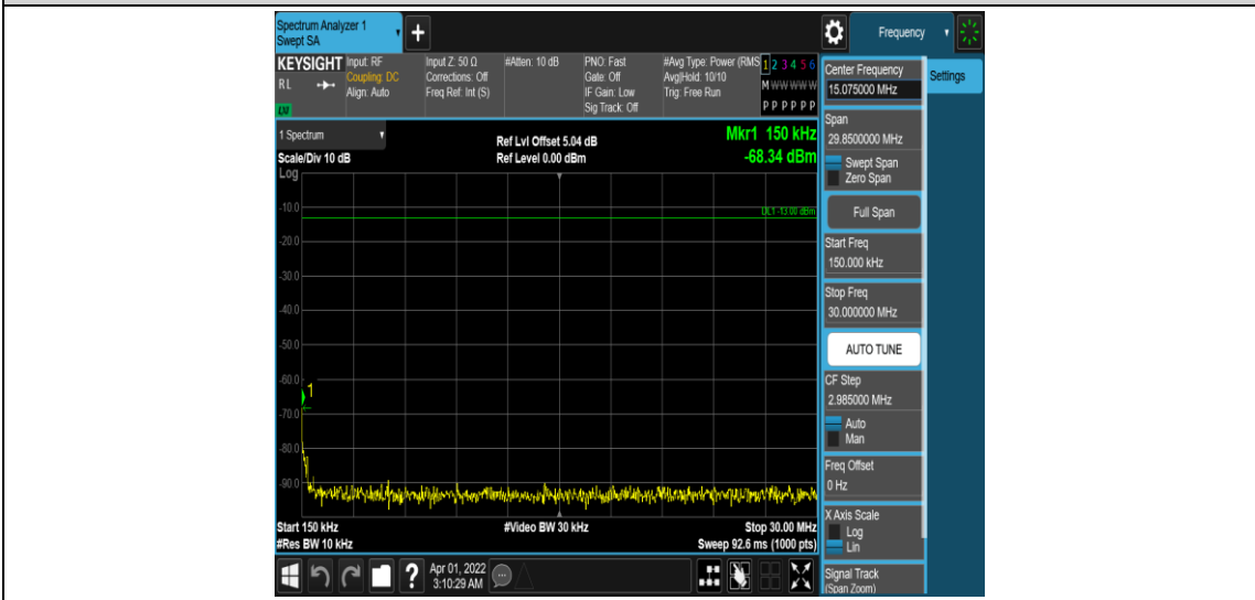
Band25-3MHz-QPSK-26675-1RB#0-Range2:0.15~30MHz
