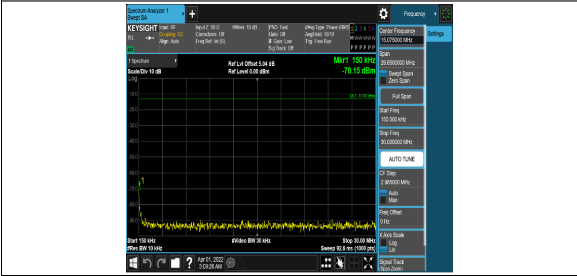
Band25-3MHz-16QAM-26365-1RB#0-Range2:0.15~30MHz
