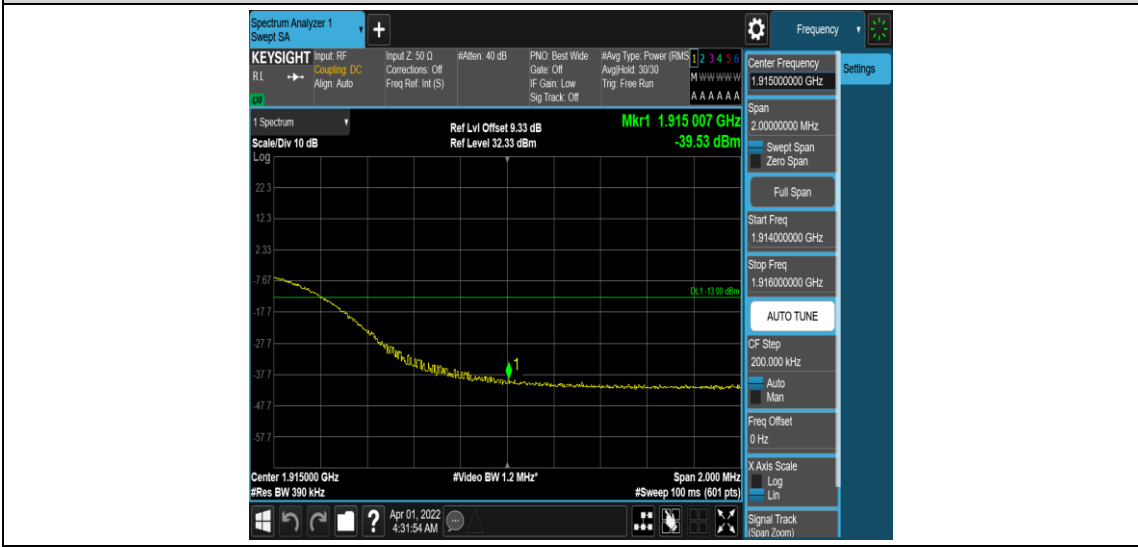
Band25-20MHz-QPSK-26590-100RB#0
