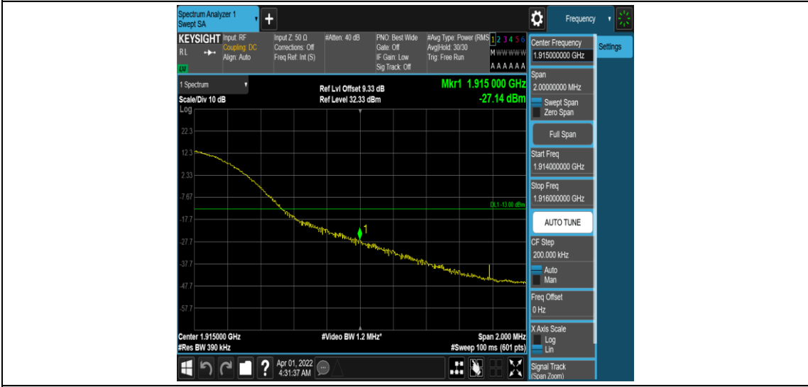
Band25-20MHz-16QAM-26590-1RB#99
