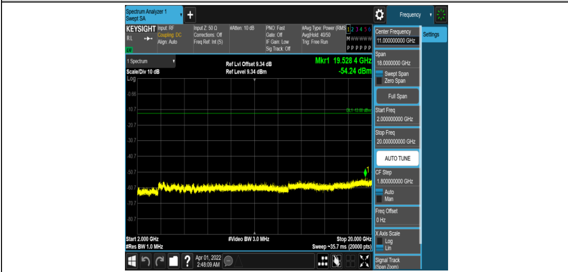
Band25-1.4MHz-QPSK-26365-1RB#0-Range5:2000~20000MHz
