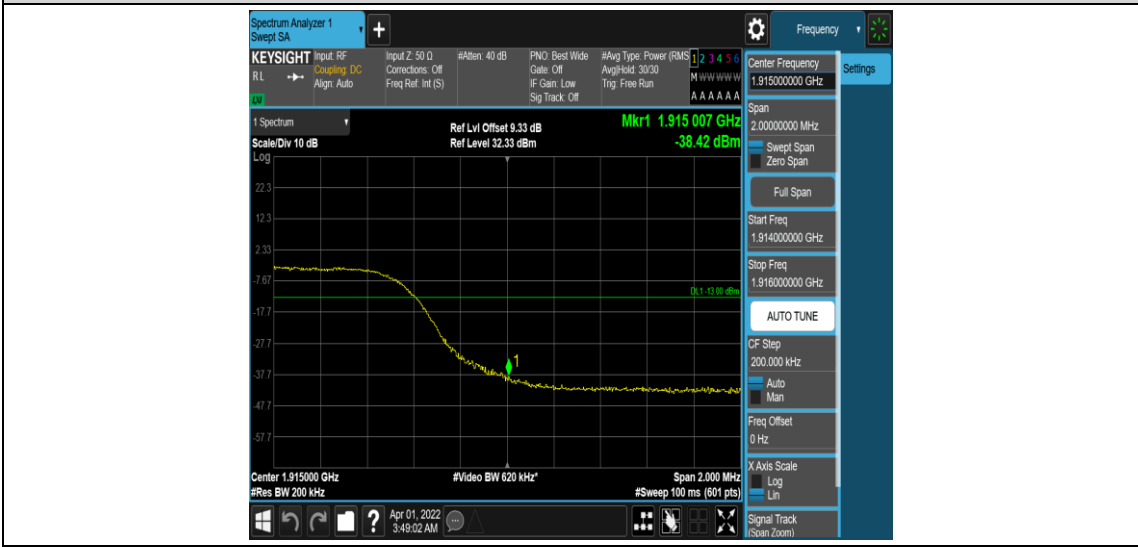
Band25-10MHz-QPSK-26640-50RB#0
