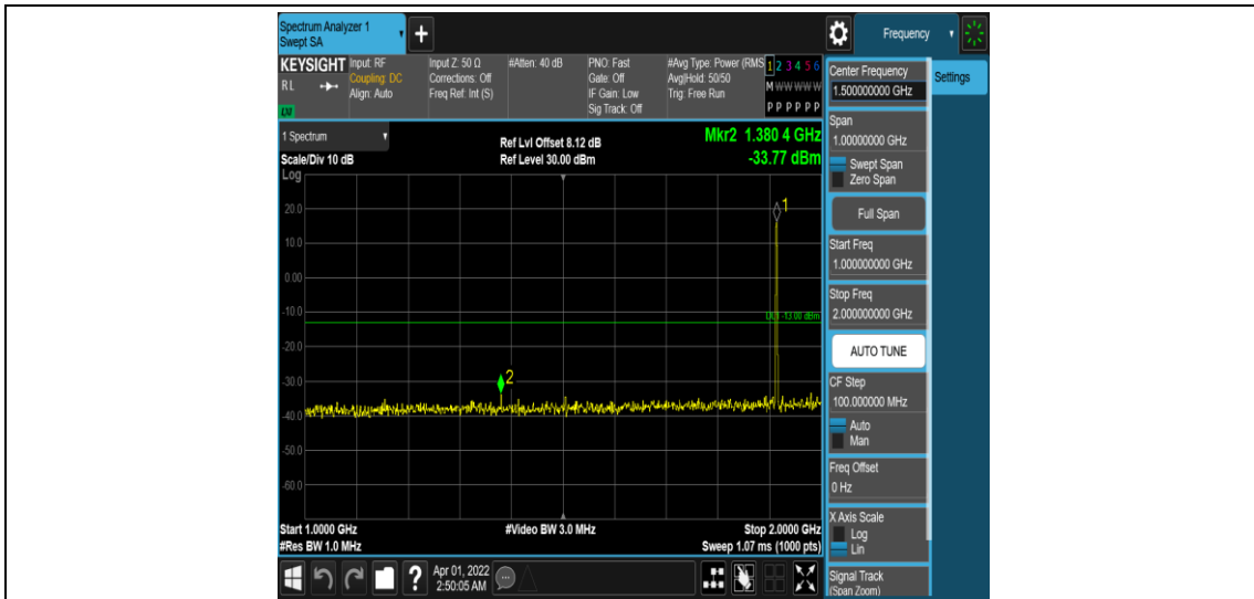
Band25-1.4MHz-QPSK-26683-1RB#0-Range4:1000~2000MHz
