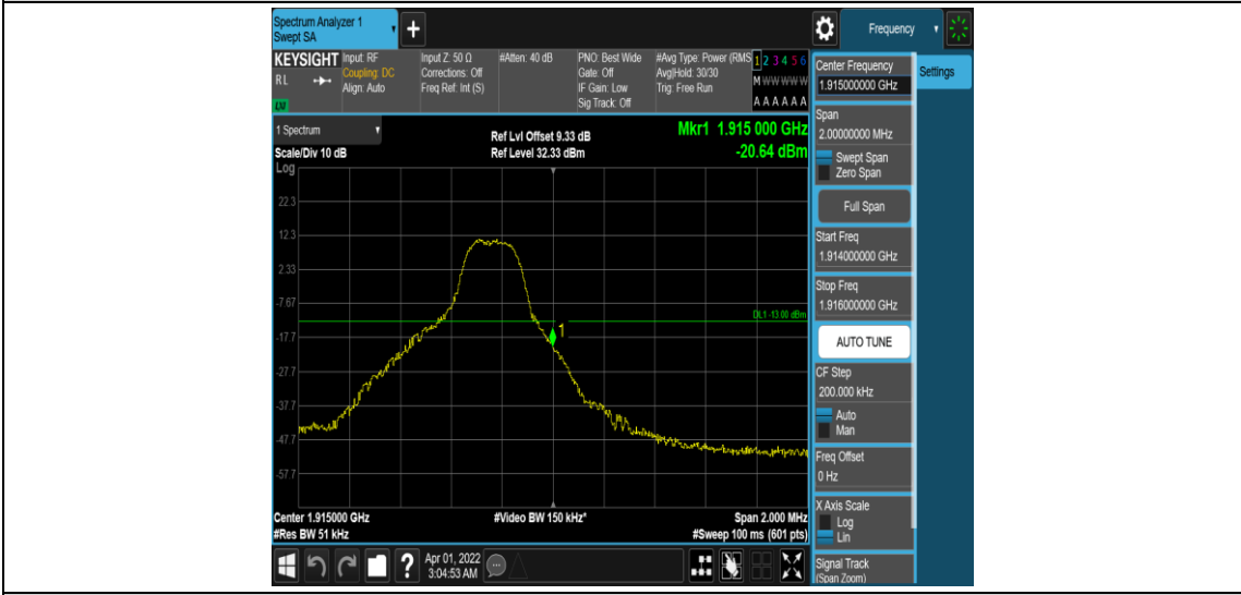
Band25-3MHz-QPSK-26675-1RB#14
