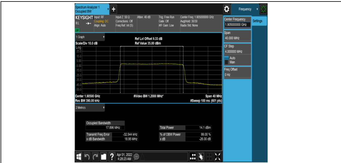
Band25-20MHz-QPSK-26590-100RB#0
