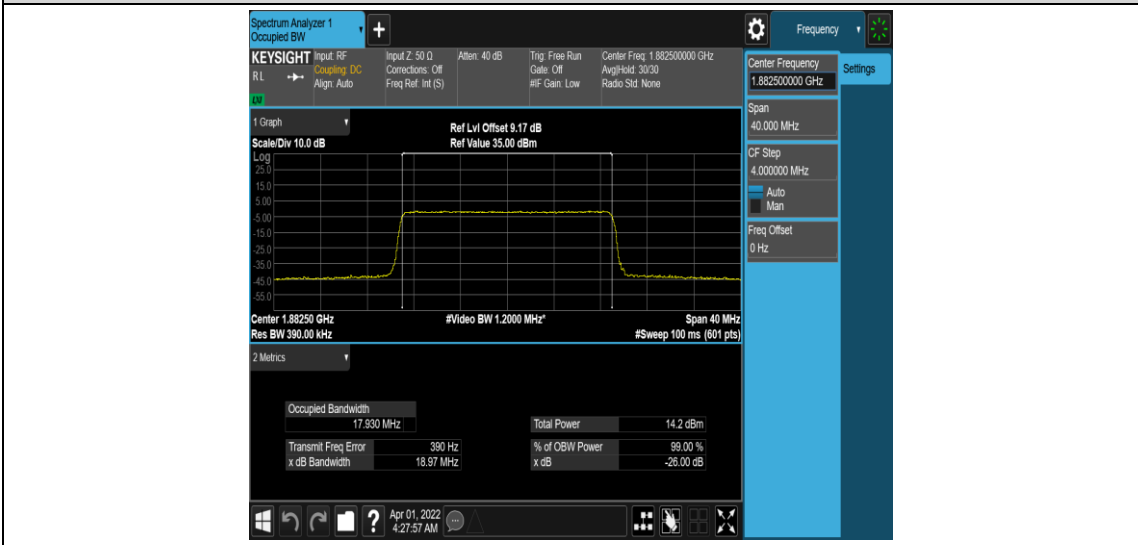
Band25-20MHz-QPSK-26365-100RB#0
