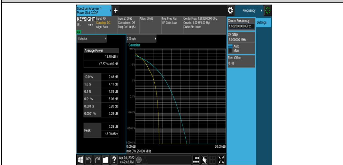
Band25-20MHz-QPSK-26365-1RB#0
