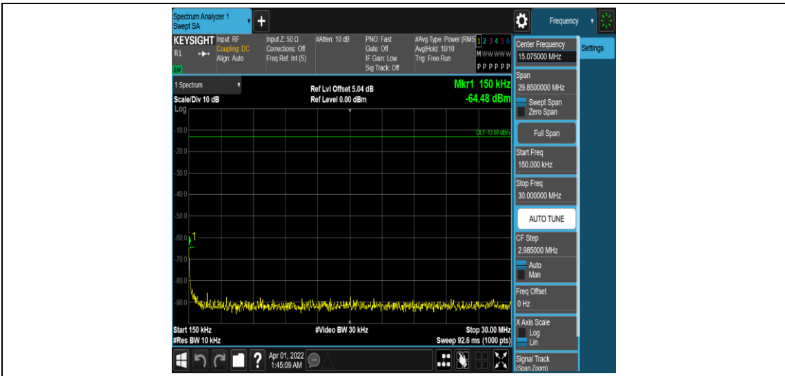
Band13-10MHz-QPSK-23230-1RB#0-Range2:0.15~30MHz
