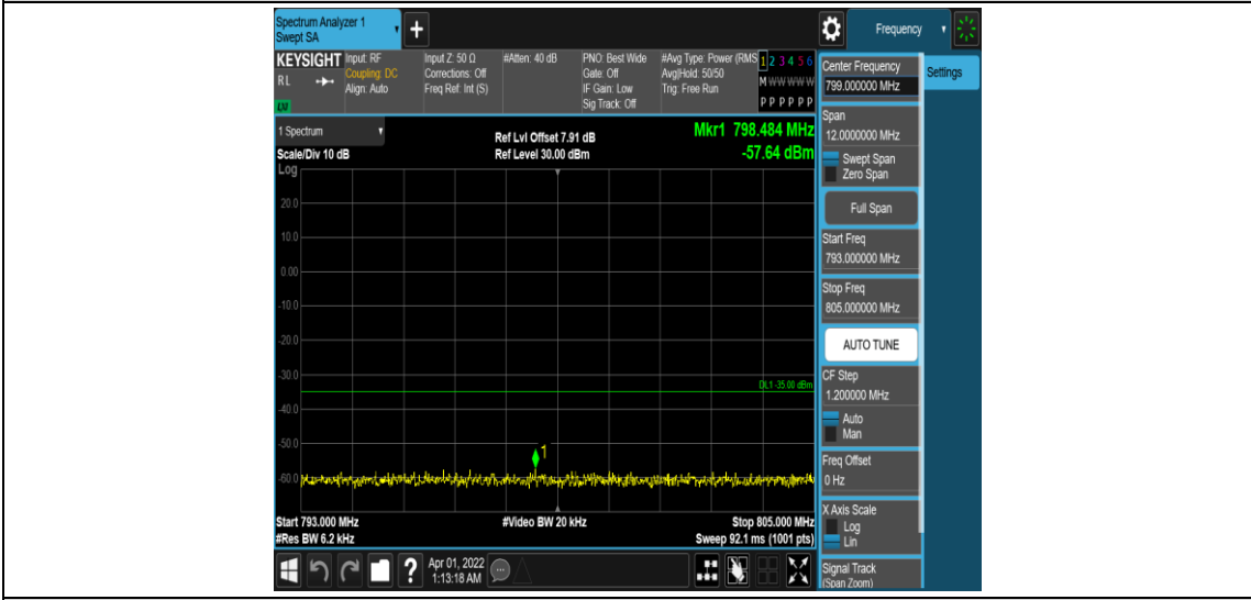
Band13-5MHz-QPSK-23230-1RB#0-Range6:793~805MHz
