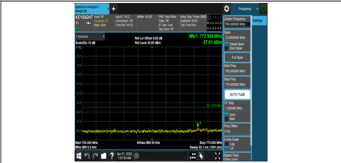
Band13-5MHz-QPSK-23205-1RB#0-Range5:763~775MHz
