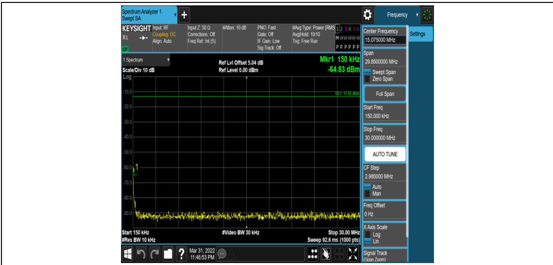
Band12-1.4MHz-16QAM-23017-1RB#0-Range2:0.15~30MHz
