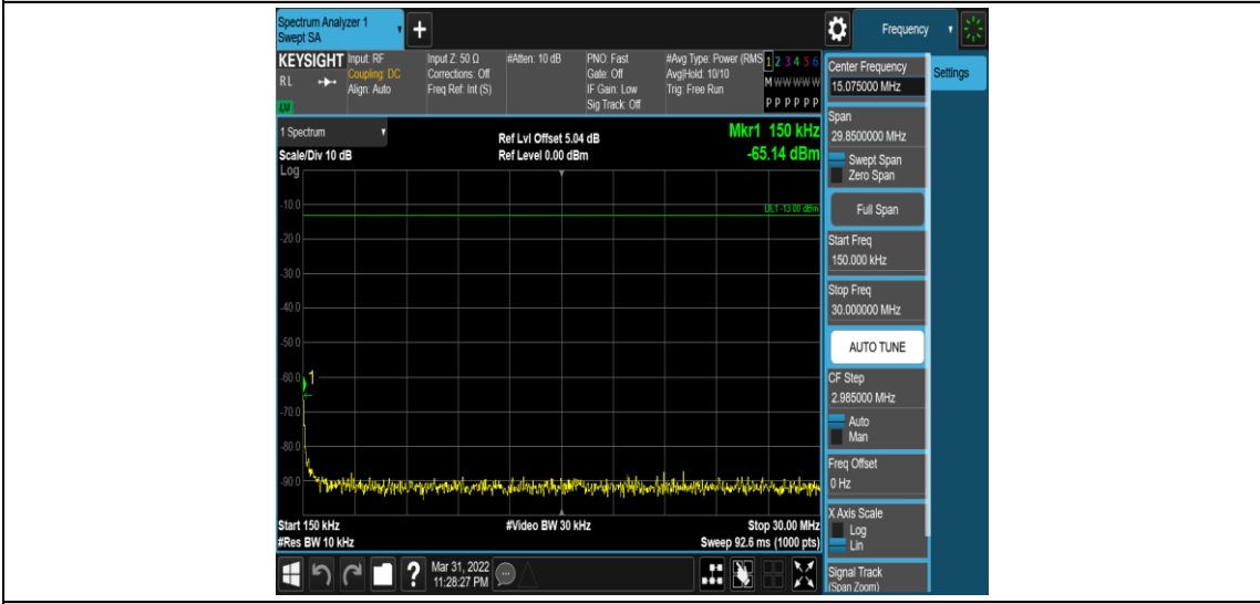
Band5-10MHz-QPSK-20525-1RB#0-Range2:0.15~30MHz
