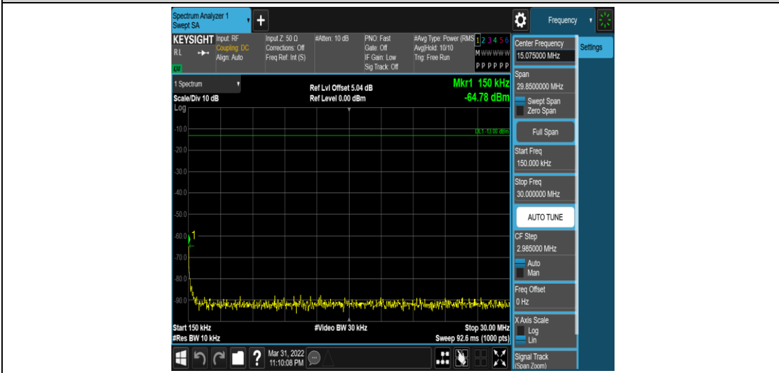
Band5-5MHz-QPSK-20625-1RB#0-Range2:0.15~30MHz
