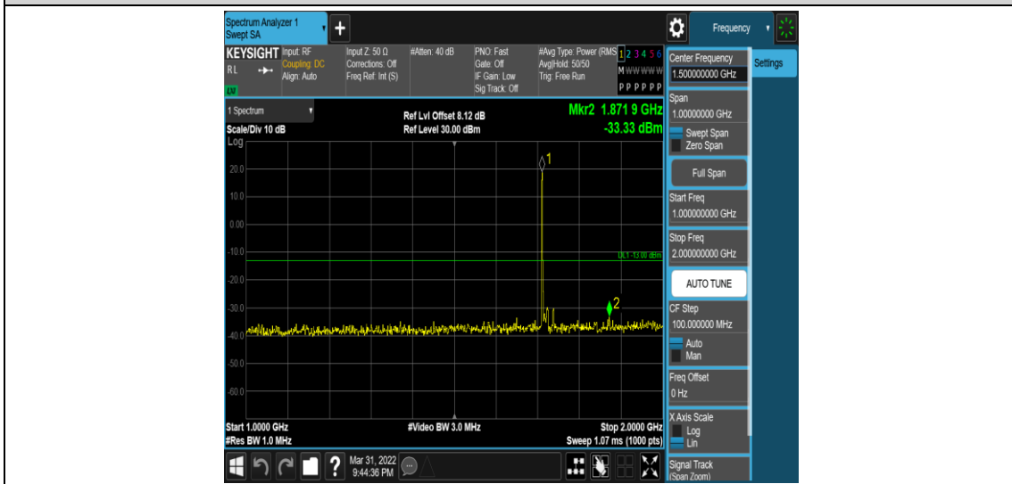
Band4-15MHz-QPSK-2025-1RB#0-Range4:1000~2000MHz
