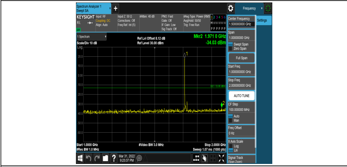
Band4-10MHz-QPSK-20000-1RB#0-Range4:1000~2000MHz
