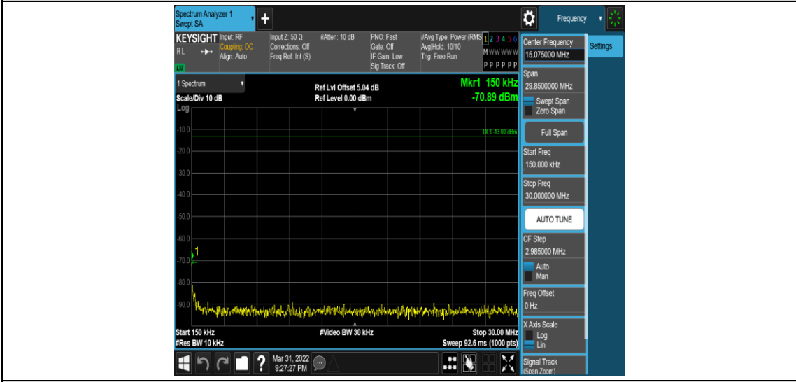
Band4-10MHz-QPSK-20350-1RB#0-Range2:0.15~30MHz
