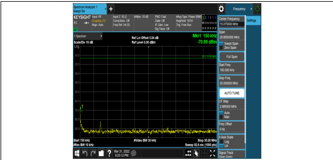
Band4-10MHz-QPSK-20000-1RB#0-Range2:0.15~30MHz
