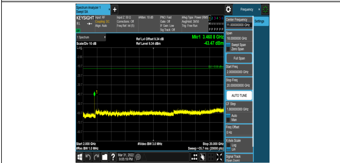
Band4-5MHz-QPSK-20175-1RB#0-Range5:2000~20000MHz
