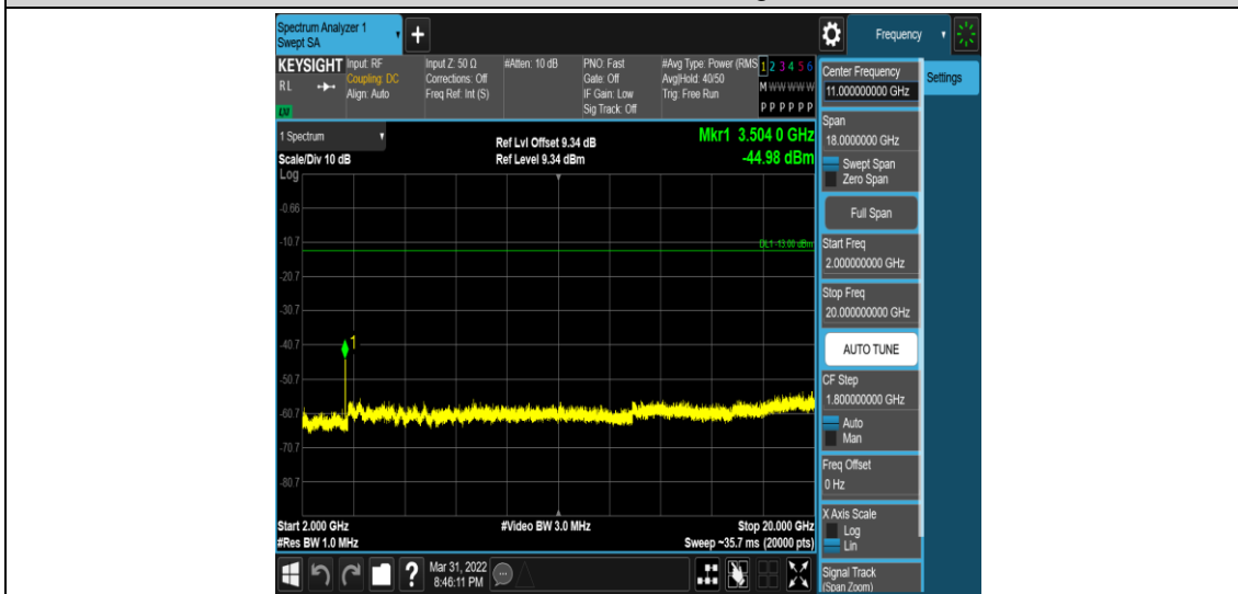
Band4-3MHz-QPSK-20385-1RB#0-Range5:2000~20000MHz
