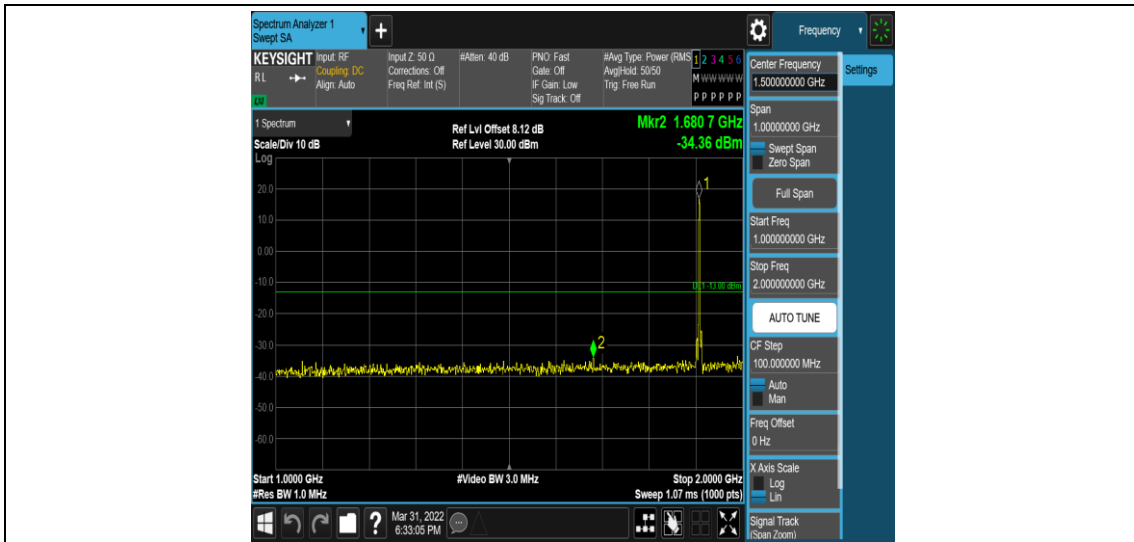
Band2-3MHz-QPSK-19185-1RB#0-Range4:1000~2000MHz
