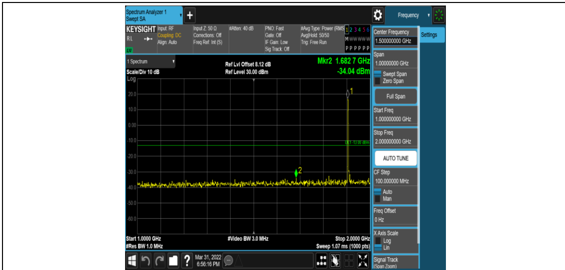
Band2-5MHz-QPSK-19175-1RB#0-Range4:1000~2000MHz
