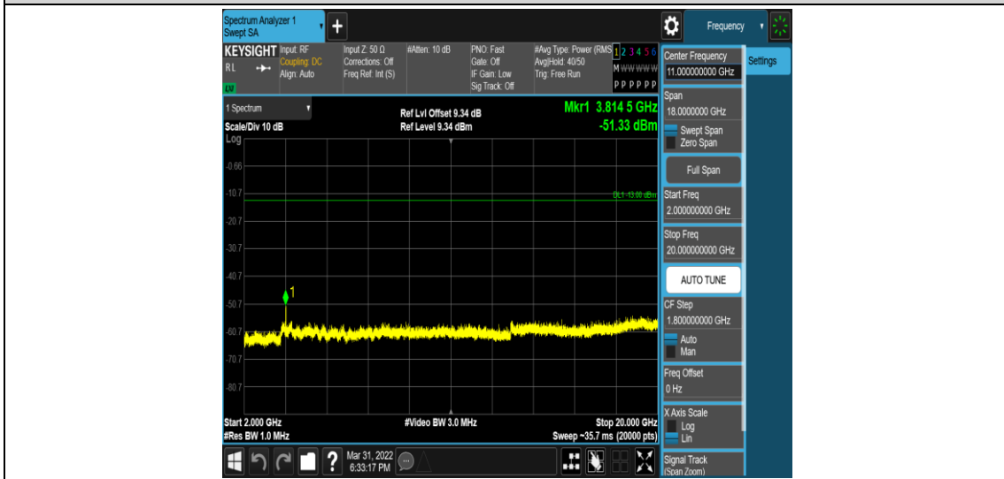
Band2-3MHz-QPSK-19185-1RB#0-Range5:2000~20000MHz
