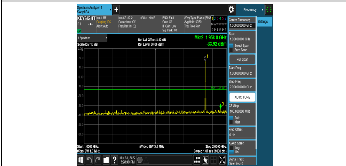
Band2-3MHz-QPSK-18615-1RB#0-Range4:1000~2000MHz
