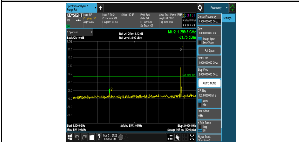
Band2-3MHz-QPSK-18900-1RB#0-Range4:1000~2000MHz
