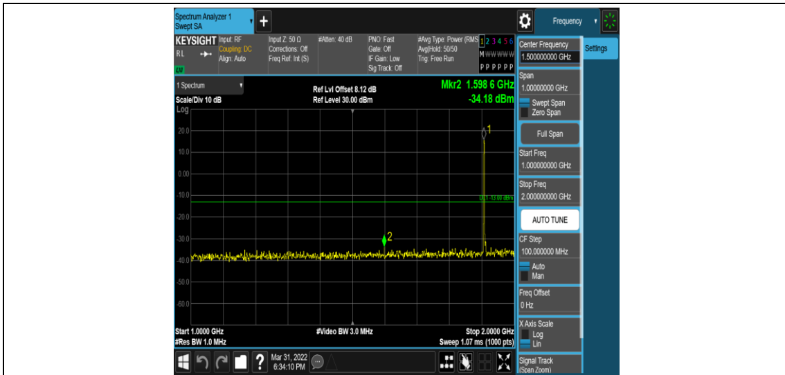
Band2-3MHz-16QAM-19185-1RB#0-Range4:1000~2000MHz
