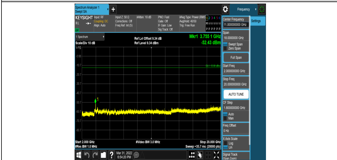
Band2-5MHz-QPSK-18900-1RB#0-Range5:2000~20000MHz
