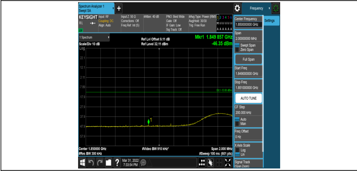
Band2-15MHz-QPSK-18675-1RB#74
