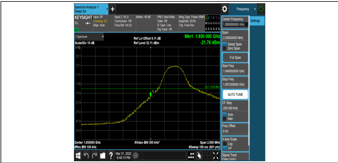
Band2-5MHz-16QAM-18625-1RB#0
