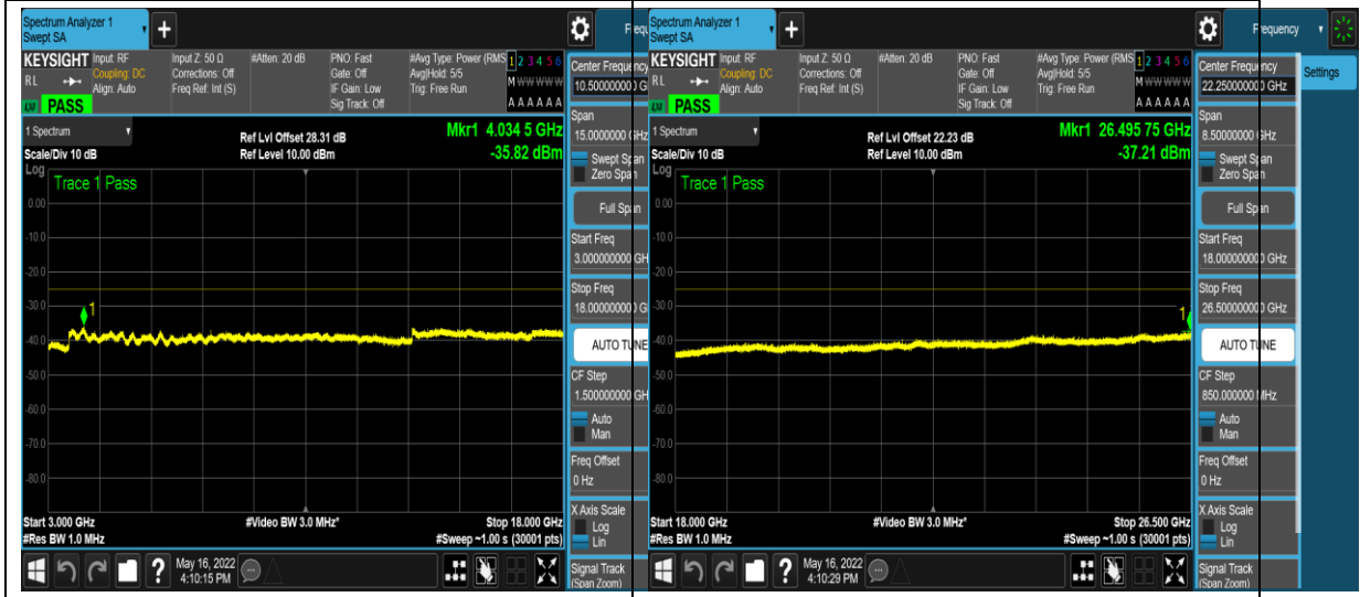
1-N41-PC3-30-90-L-16-CP-QPSK-Edge_1R B_Left-1@0-30-1000--68.99--35-PASS
