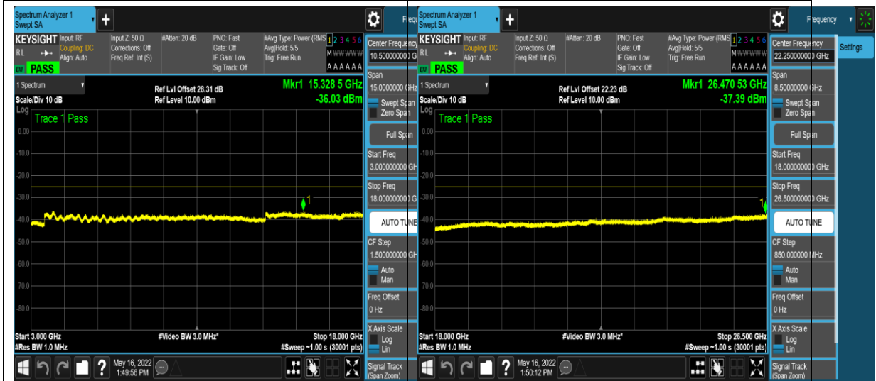
1-N41-PC3-30-40-M-4-DFT-QPSK-Edge_1R B_Left-1@0-3000-18000--36.03--25-PASS
