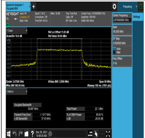
n41-PC3-30-40-H-3-N/A-N/A-N/A-DFT-16QA M-Outer_Full-100@0-Ant1-35.687-37.40-≤40 -PASS
