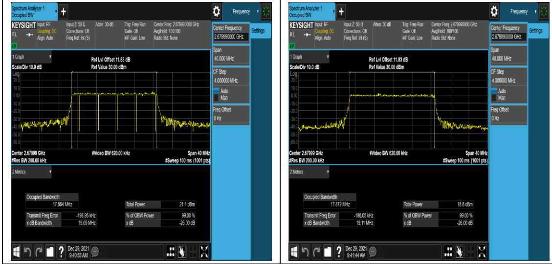
n41A-PC3-30-20-H-3-N/A-N/A-N/A-DFT-16Q AM-Outer_Full-50@0-Ant1-17.864-19.09-≤20 -PASS
