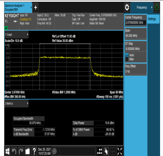
n41-PC3-30-40-H-4-N/A-N/A-N/A-DFT-64QA M-Outer_Full-100@0-Ant1-35.678-37.67-≤40 -PASS
