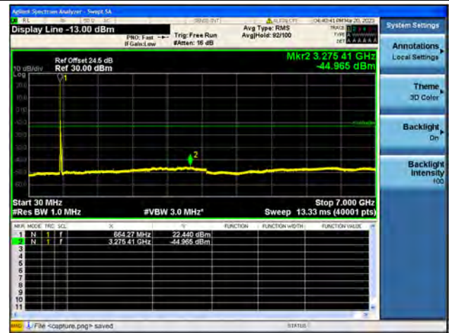
Band71 / 20MHz / Low CH / QPSK
