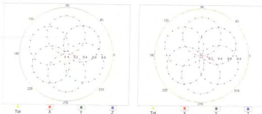
f=1800 MHz,R22
