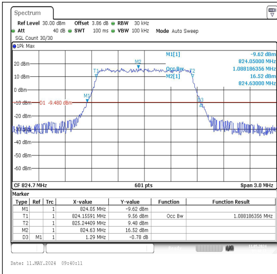
26(824-849)-1.4MHz-QPSK-26797-6RB#0-PASS
