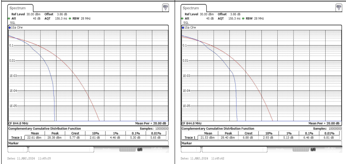
26(824-849)-10MHz-QPSK-26990-1RB#0-PASS 26(824-849)-10MHz-16QAM-26990-1RB#0-PASS
