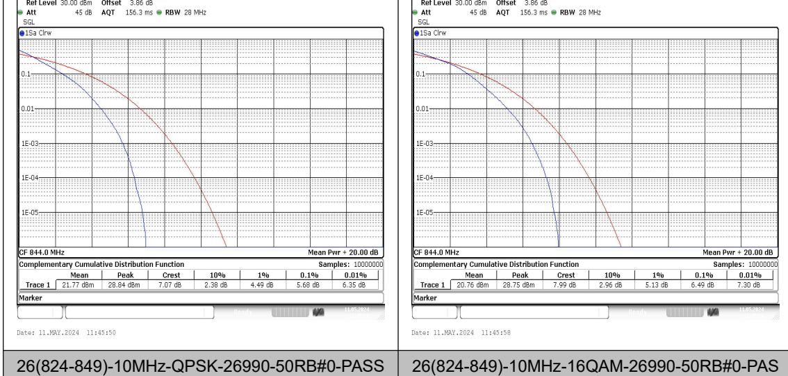
26(824-849)-10MHz-QPSK-26990-50RB#0-PASS 26(824-849)-10MHz-16QAM-26990-50RB#0-PAS
