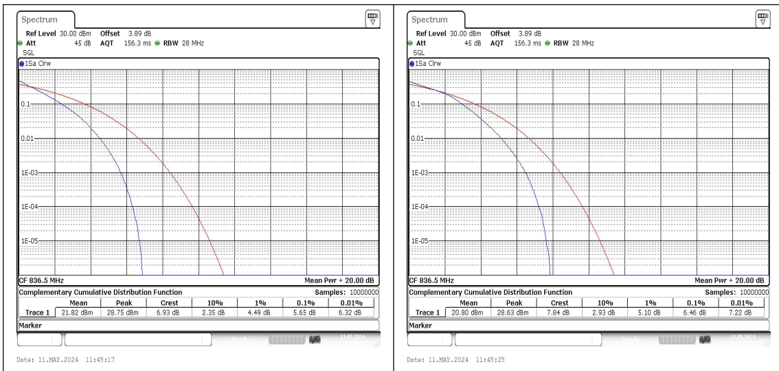
26(824-849)-10MHz-QPSK-26915-50RB#0-PASS 26(824-849)-10MHz-16QAM-26915-50RB#0-PAS
