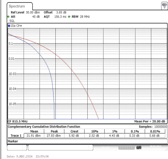
26(814-824)-3MHz-QPSK-26705-15RB#0-PASS
