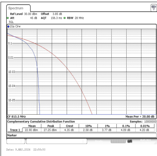
26(814-824)-3MHz-QPSK-26705-1RB#0-PASS
