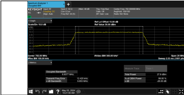
Band 13 23230/782.0/Mid QPSK 50@0
