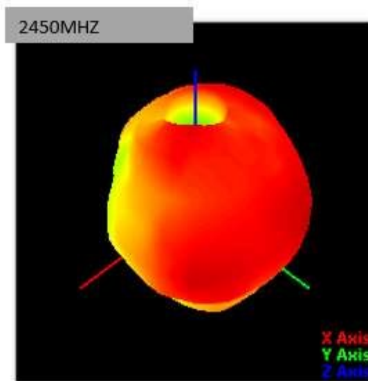
WIFI/BT 辐射方向图 Radiation Patterns
