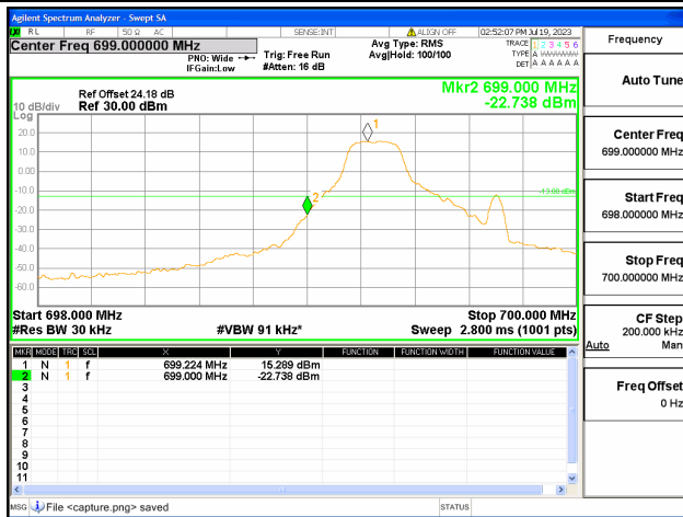
B12 / 1.4MHz / Low CH / QPSK / 1 RB
