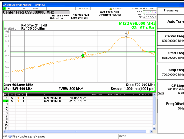
B12 / 10MHz / Low CH / QPSK / 1 RB
