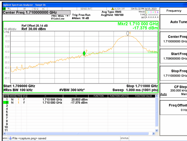
B66 / 10MHz / Low CH / QPSK / 1 RB
