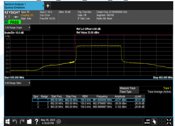
B71_10M_16QAM_50@0_CH_133172
