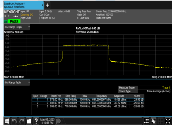
B71_10M_QPSK_50@0_CH_133422
