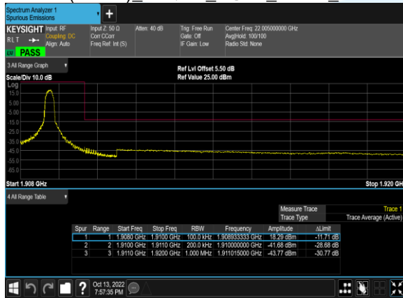
B2(20.0M)_16QAM_1@99_19100_CH
