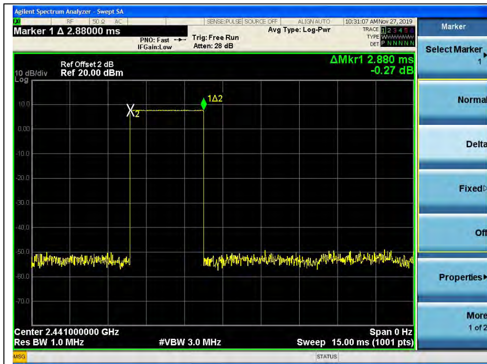
(DH5, GFSK)
