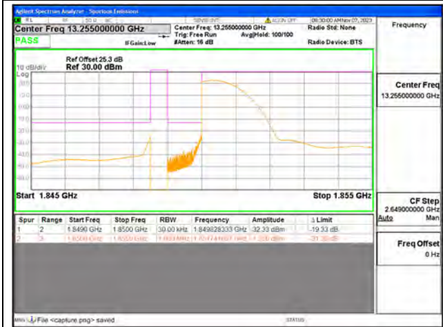
B2 / 5MHz / Low CH / QPSK / 1 RB
