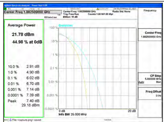
B25 / 20MHz / Mid CH / 16QAM
