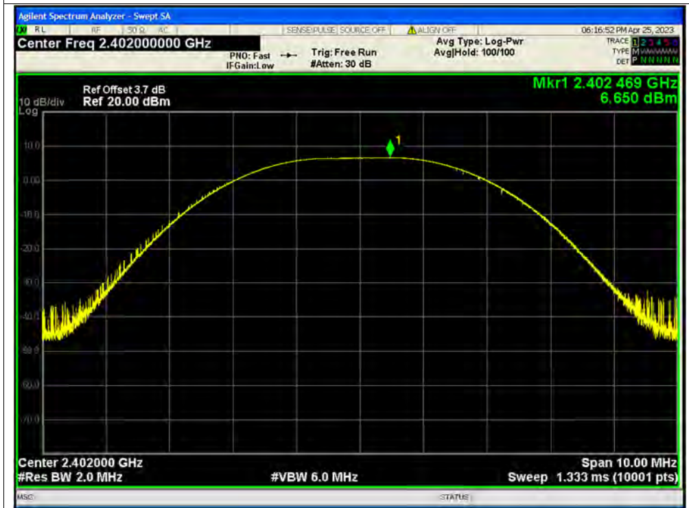
Peak Power NVNT BLE 2M 2402MHz Ant1
