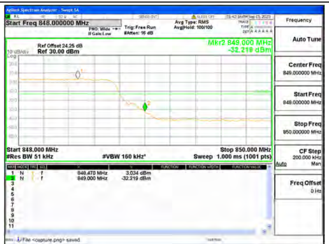
B5 / 5MHz / High CH / QPSK / FULL RB
